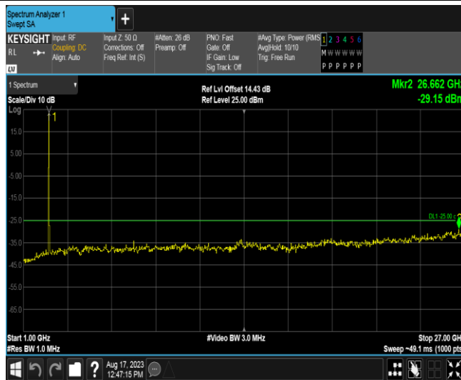
Band41-20MHz-16QAM-39750-1RB#0-Range2:1000~27000MHz
