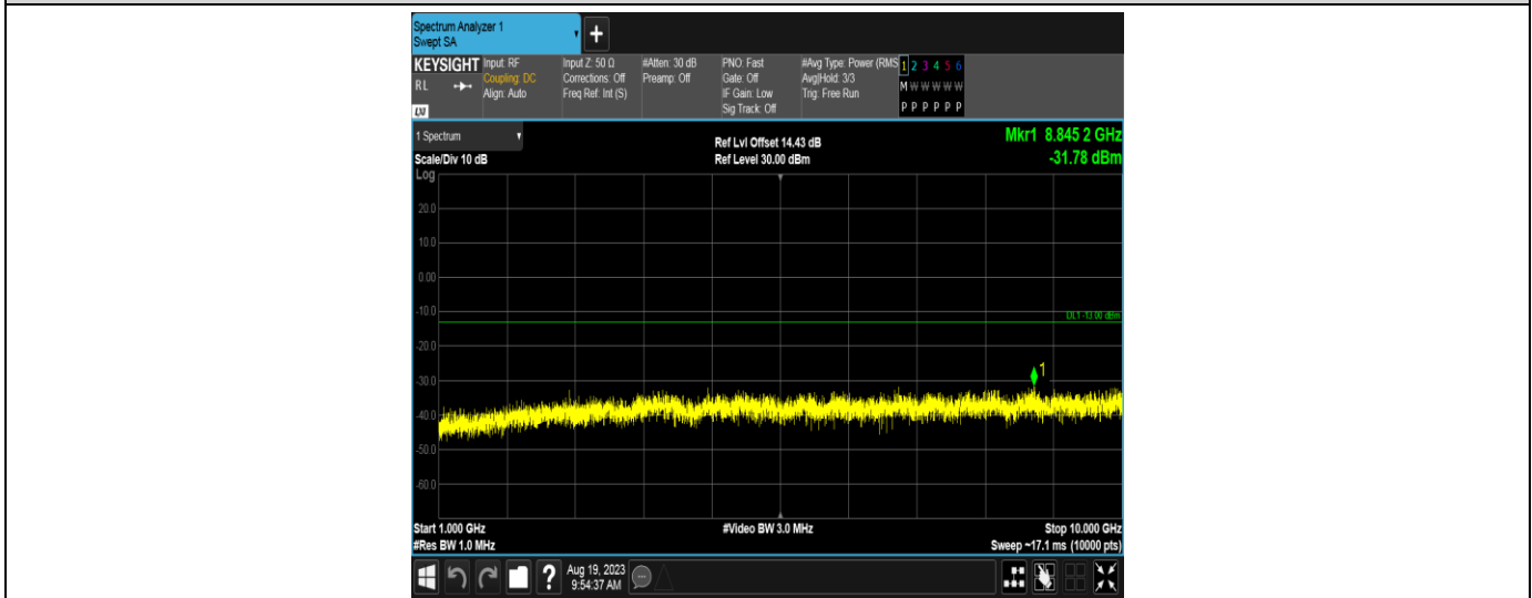
Band5-3MHz-QPSK-20415-1RB#0-Range2:1000~10000MHz
