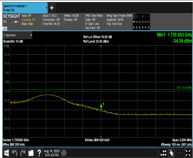
Band4-10MHz-QPSK-20350-1RB#0
