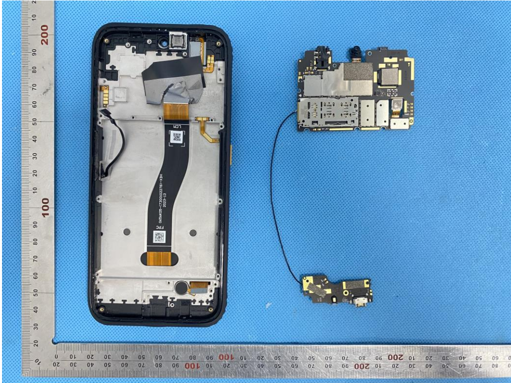
BT&WIFI&GPS&DIVERSITY ANTENNA
