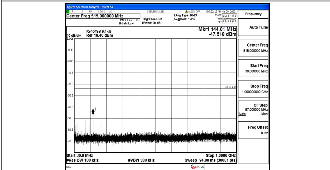
11B_Ant1_2412_30~1000
