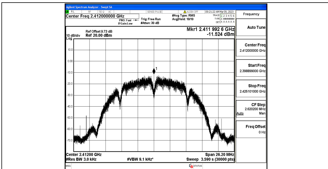
11B_Ant1_2412
