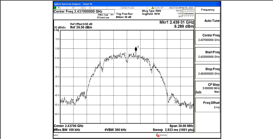
11B_Ant1_2437_0~Reference
