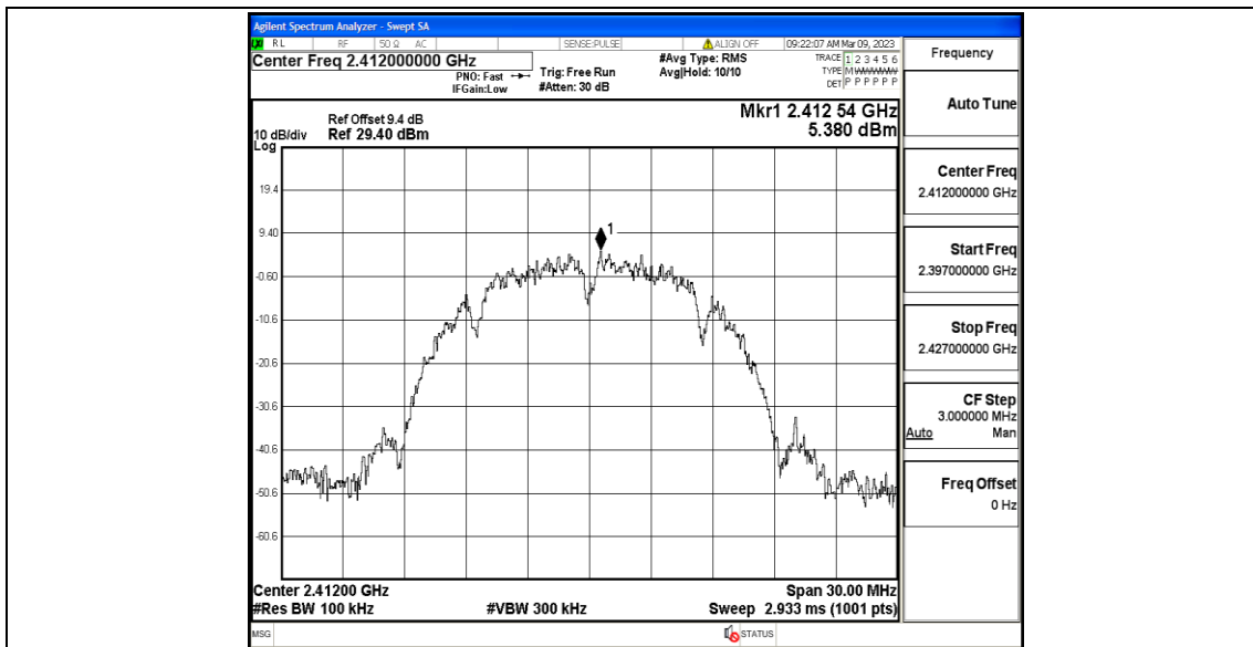
11B_Ant1_2412_0~Reference
