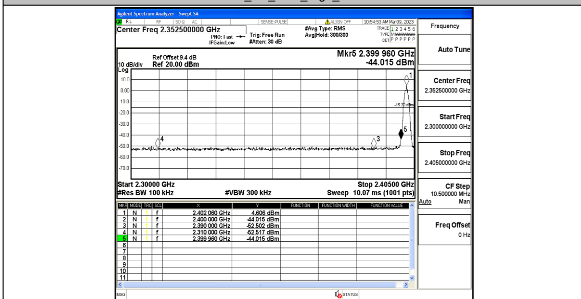
BLE_2M_Ant1_Low_2402
