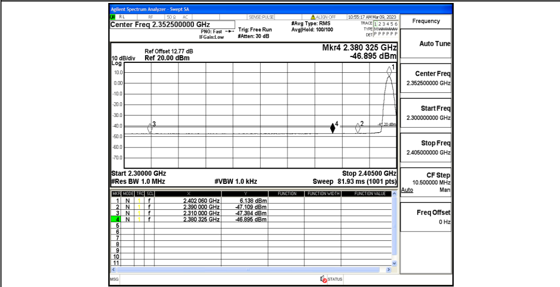
BLE_2M_Ant1_Low_2402_AV
