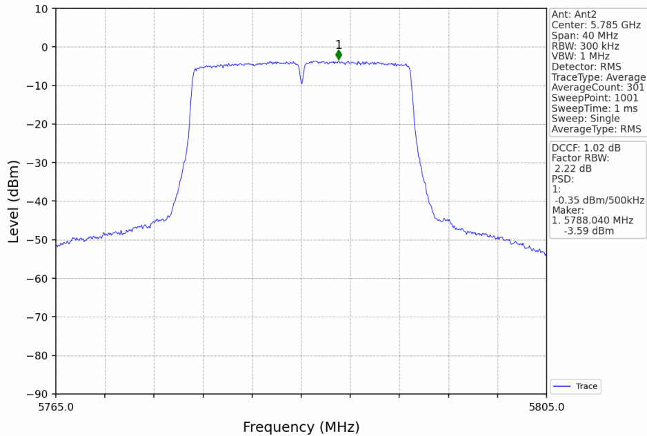
802.11n(HT20)_MCH_5785MHz_MIMO_NTNV
