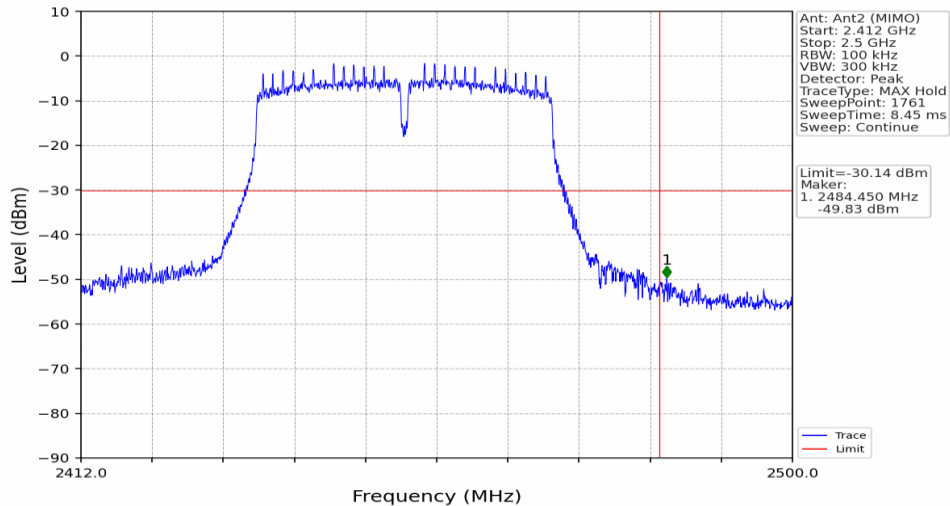
802.11n(HT40)_HCH_2452MHz_Ant2 (MIMO)_NTNV
