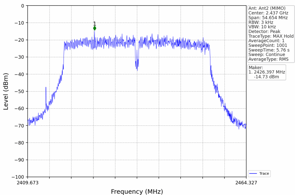
802.11n(HT40)_MCH_2437MHz_Ant2 (MIMO)_NTNV
