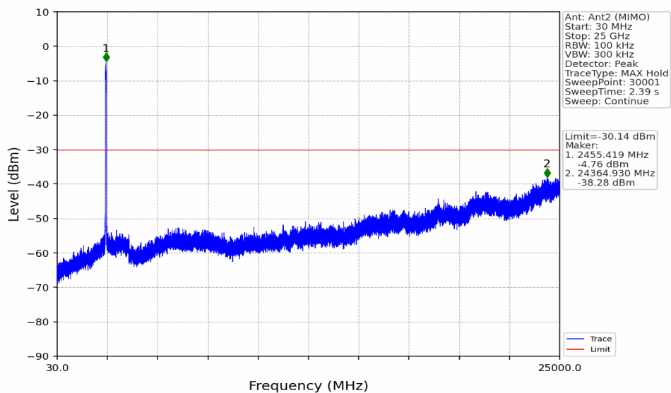
802.11n(HT40)_HCH_2452MHz_Ant2 (MIMO)_NTNV
