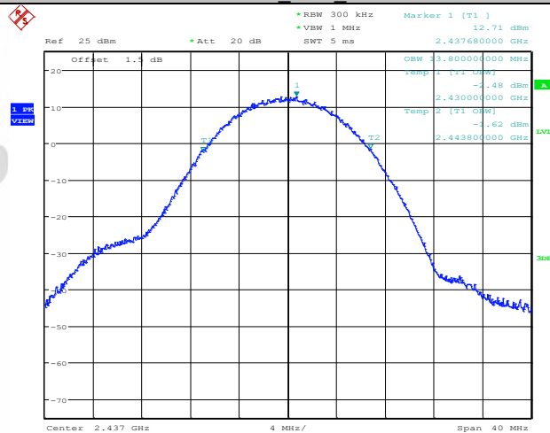
11b_Ant2_2437
