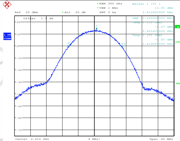
11b_Ant2_2412
