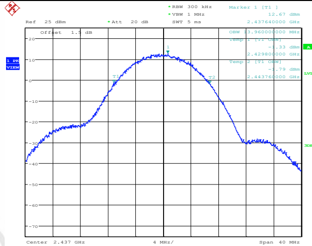
11b_Ant1_2437
