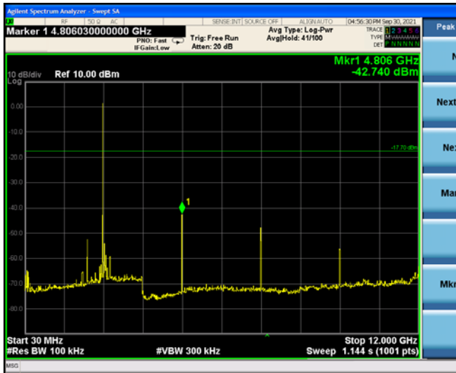
30MHz-12GHz
