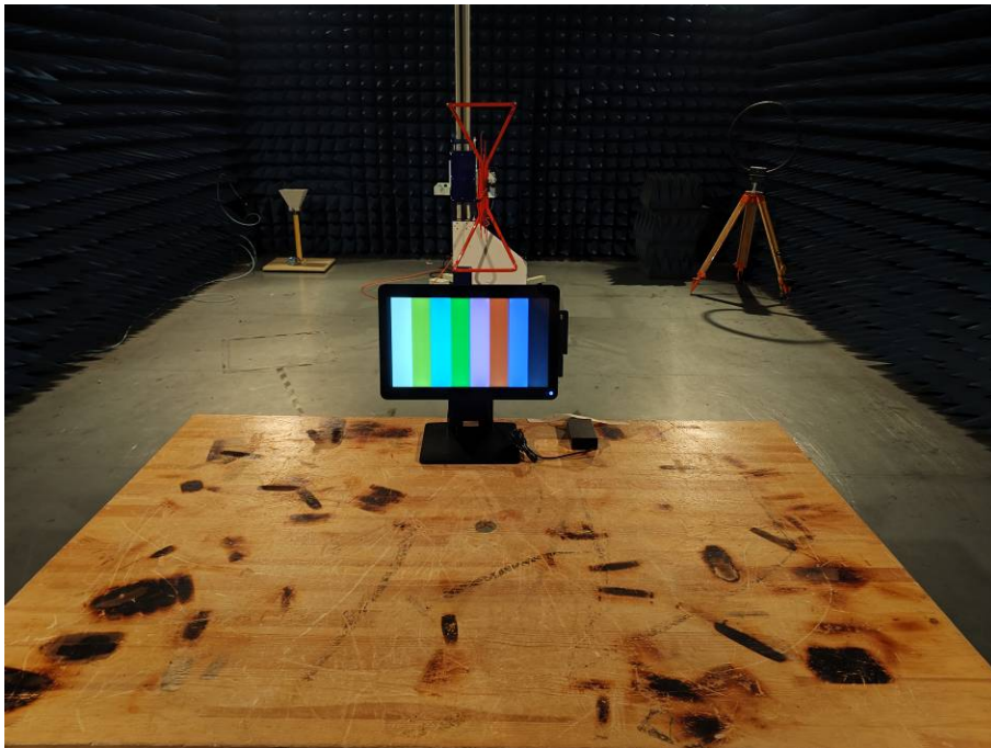
(Adapter:FSP120-AAAN3)
