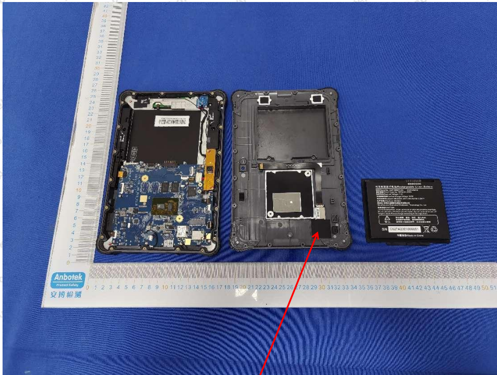
NFC ANT
