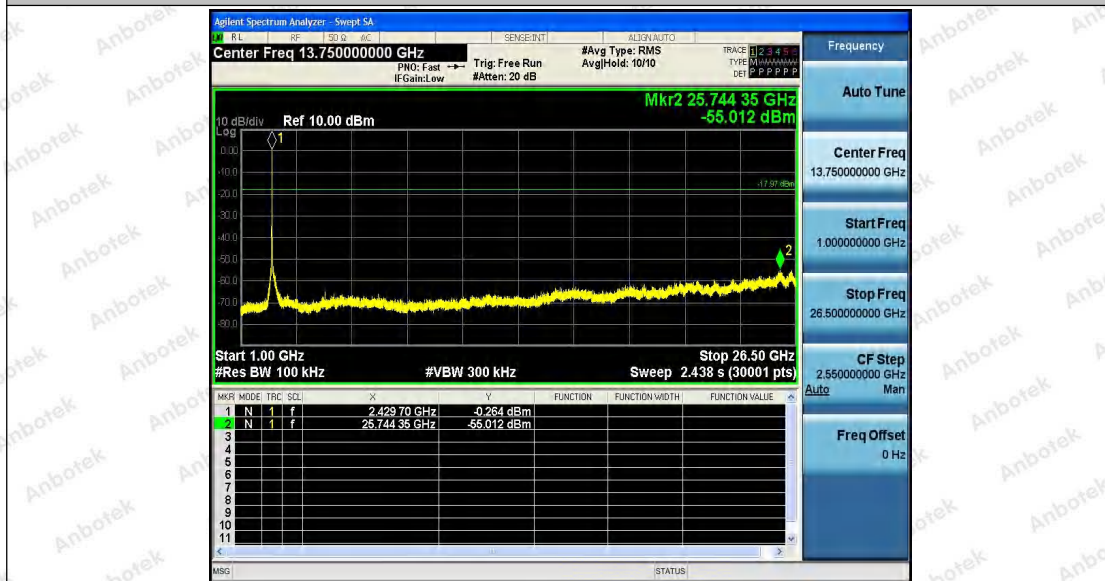
11N20_Ant1_2437_1000~26500
