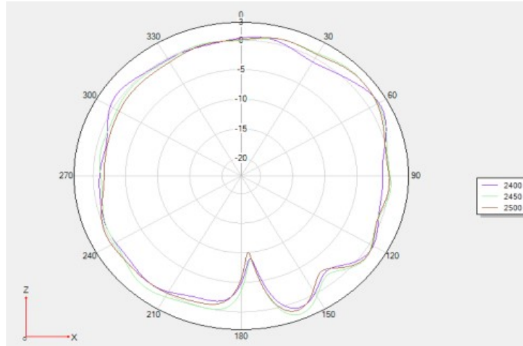
Phi 0 2D 图
