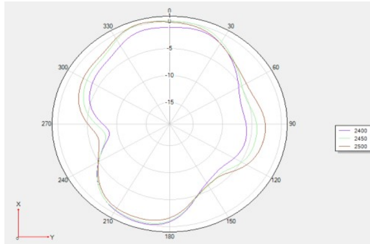
Theta 90 2D 图
