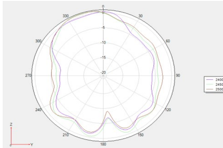
Phi 90 2D 图
