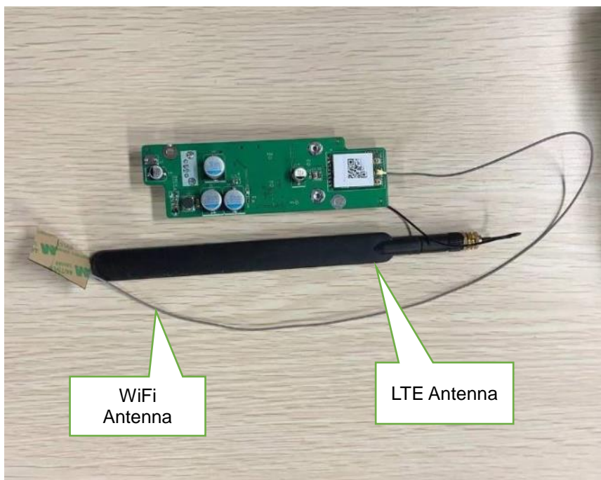
EUT Photo
