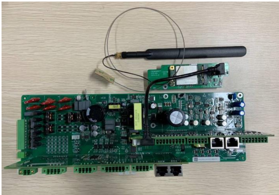
EUT Photo
