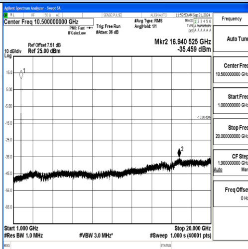
1 GHz – 20 GHz
