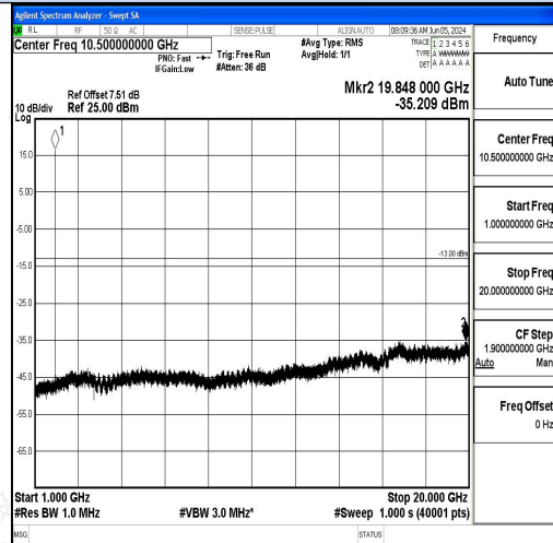
1 GHz - 20 GHz
