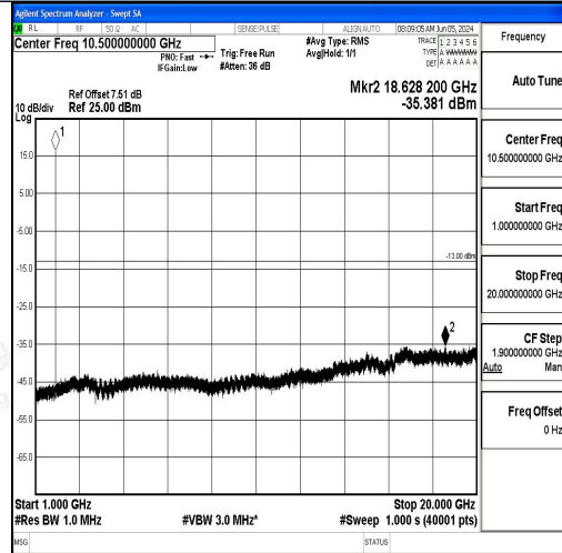
1 GHz - 20 GHz
