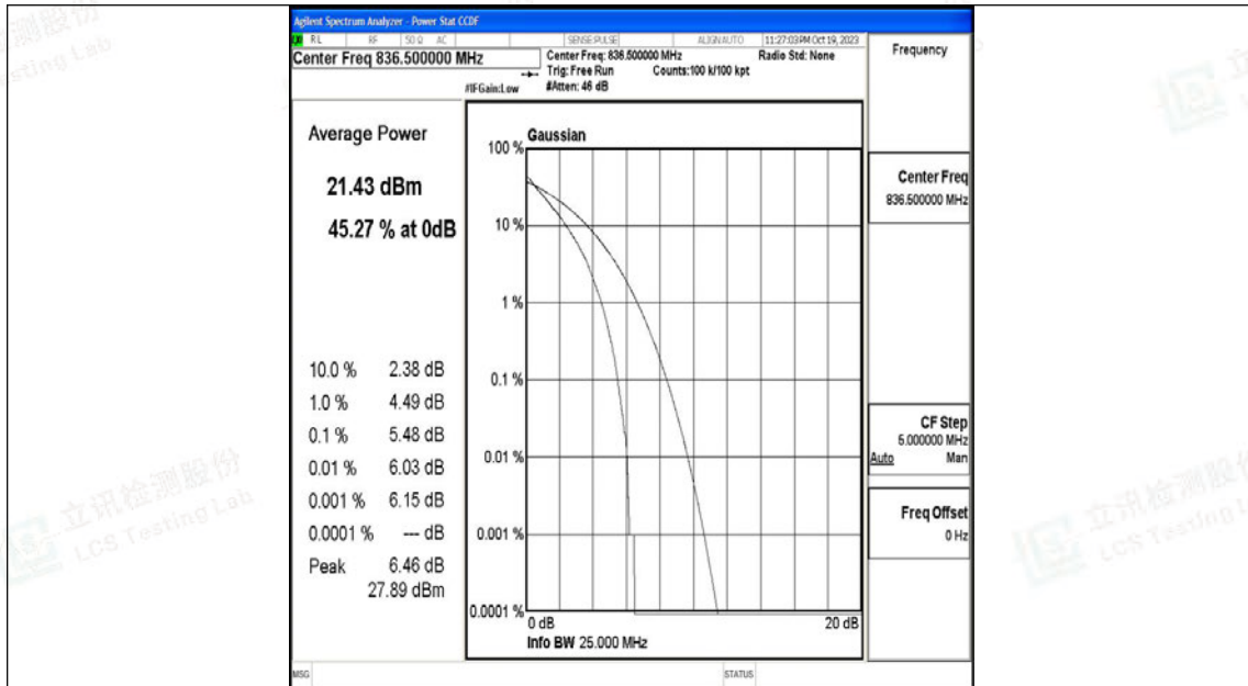
26(824-849)-10MHz-QPSK-26915-50RB#0-PASS
