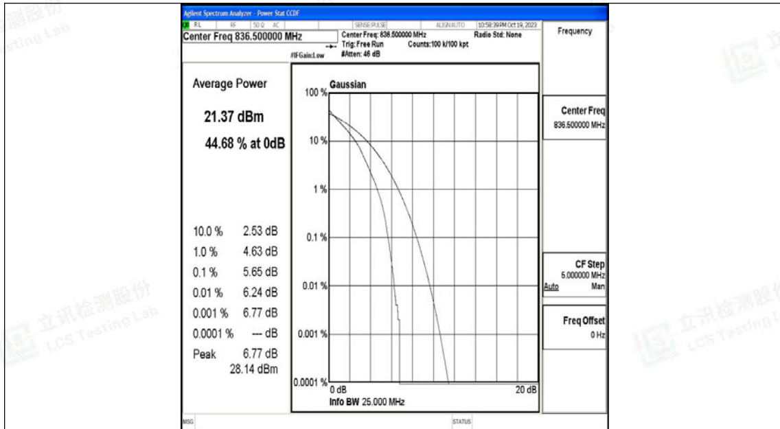
26(824-849)-3MHz-QPSK-26915-15RB#0-PASS
