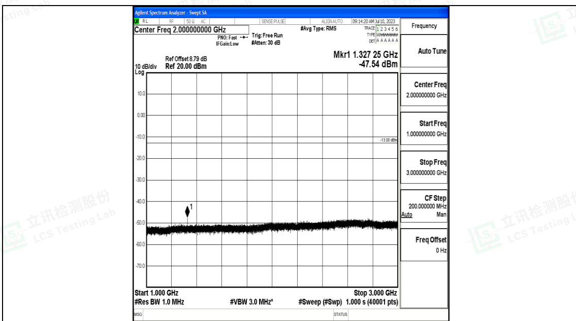
Band71_10MHz_QPSK_133172_1RB#0_1000~3000_1000~3000
