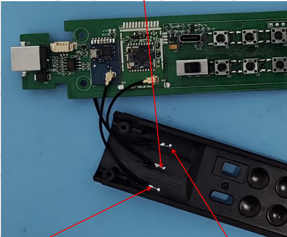
2.4G RX ANT
