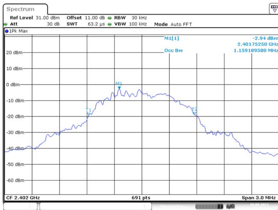
99% Bandwidth, BLE Low Channel
