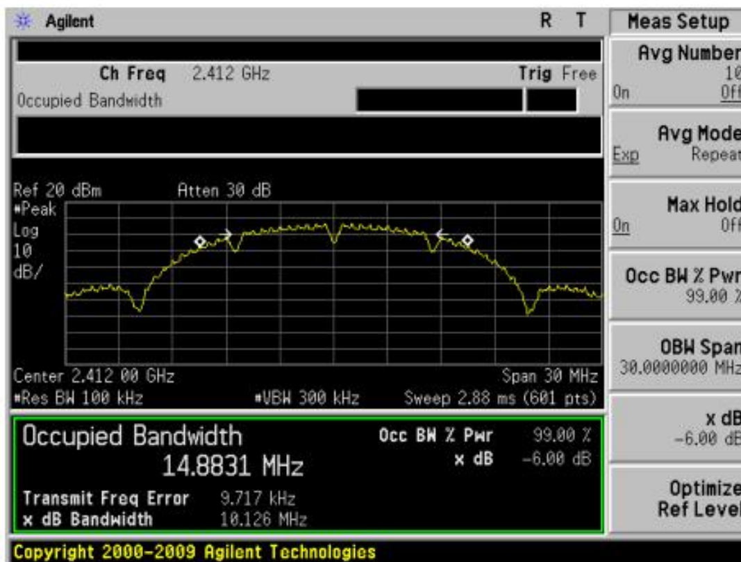
802.11b-CH2412MHZ
