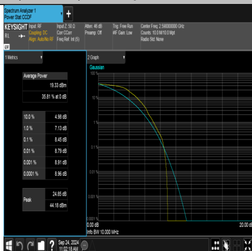
Band41(2535-2655)-10MHz-QPSK-40590-1RB#0-PASS
