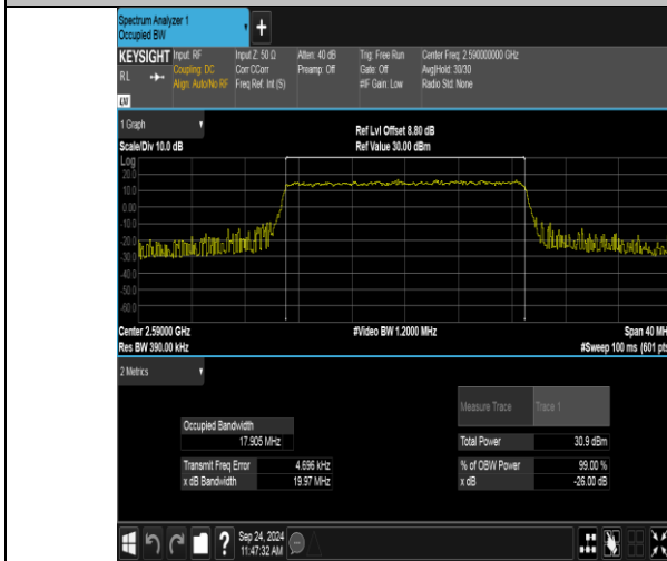
Band41(2535-2655)-20MHz-QPSK-40590-100RB#0-PASS
