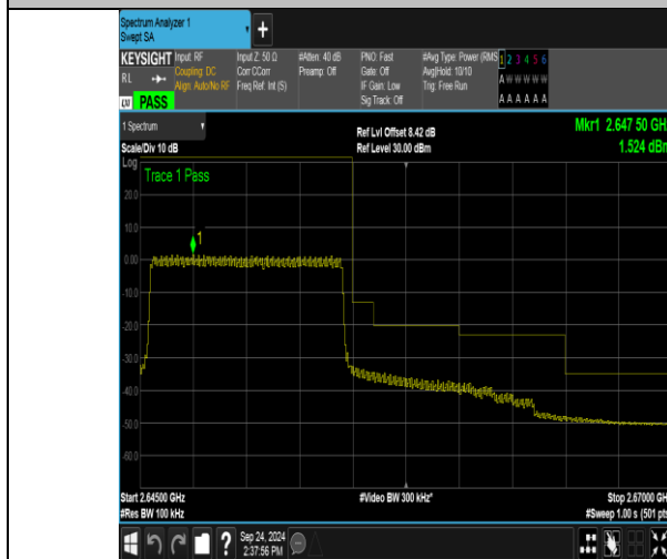
Band41_10MHz_QPSK_41190_50RB#0
