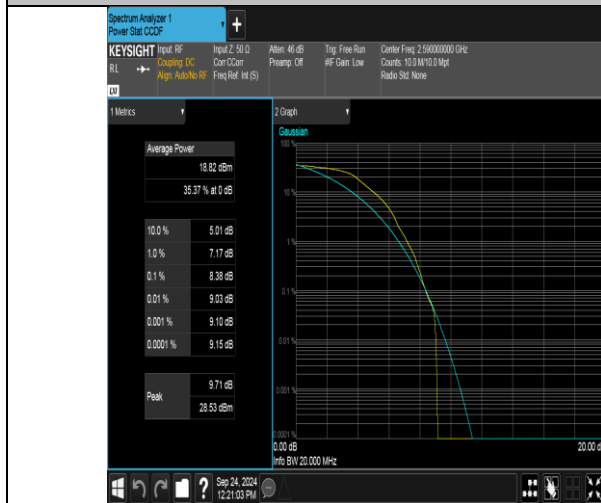
Band41(2535-2655)-20MHz-QPSK-40590-1RB#0-PASS
