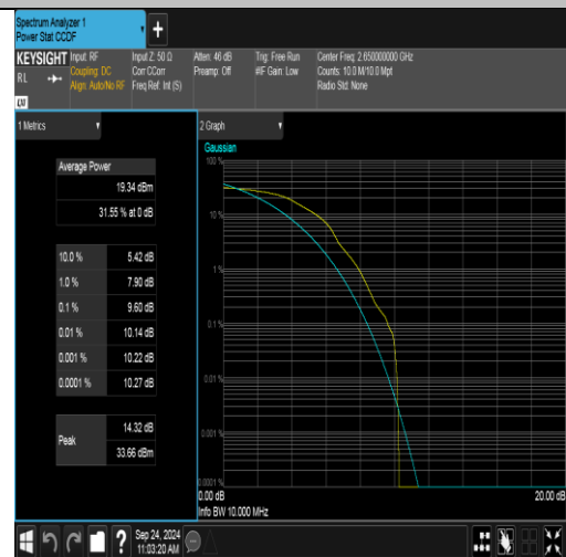
Band41(2535-2655)-10MHz-16QAM-41190-1RB#0-PASS
