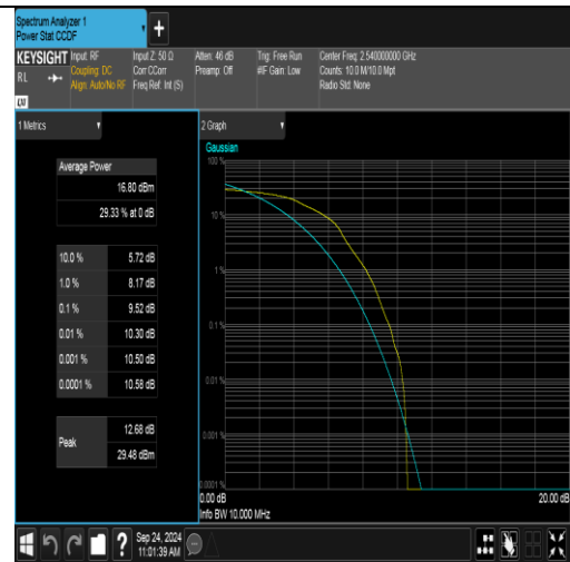
Band41(2535-2655)-10MHz-16QAM-40090-1RB#0-PASS
