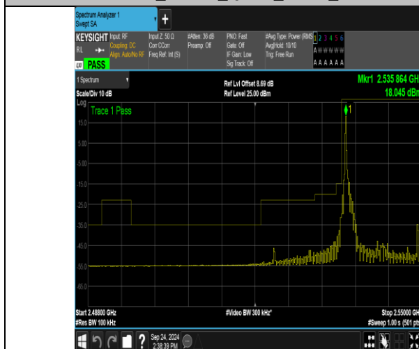
Band41_15MHz_QPSK_40115_1RB#0
