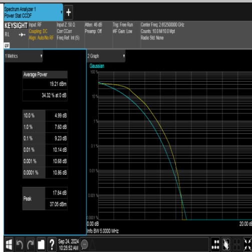
Band41(2535-2655)-5MHz-QPSK-41215-25RB#0-PASS
