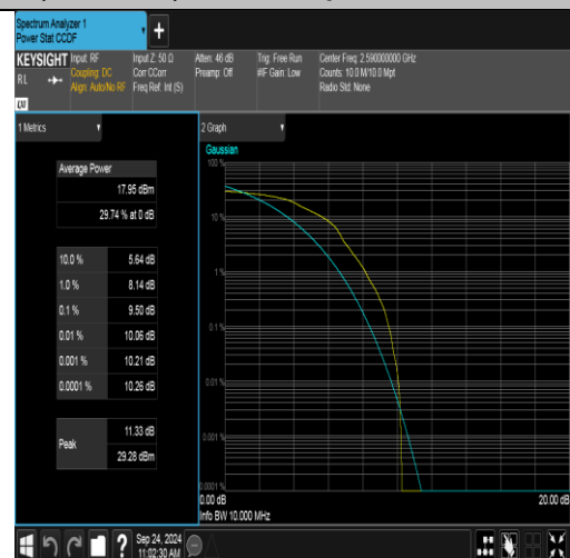
Band41(2535-2655)-10MHz-16QAM-40590-1RB#0-PASS
