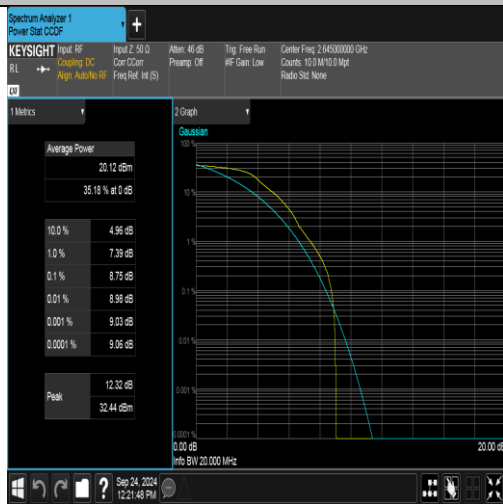
Band41(2535-2655)-20MHz-QPSK-41140-1RB#0-PASS
