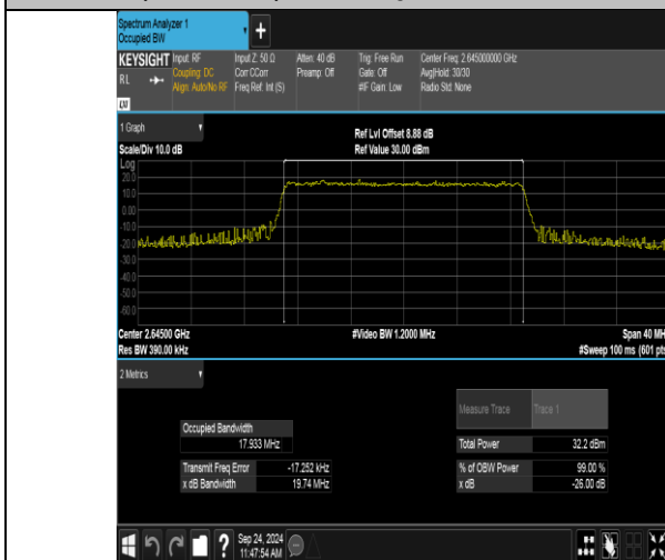
Band41(2535-2655)-20MHz-QPSK-41140-100RB#0-PASS
