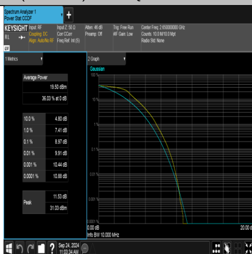
Band41(2535-2655)-10MHz-QPSK-41190-50RB#0-PASS
