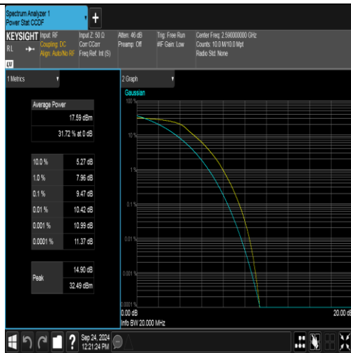
Band41(2535-2655)-20MHz-QPSK-40590-100RB#0-PASS
