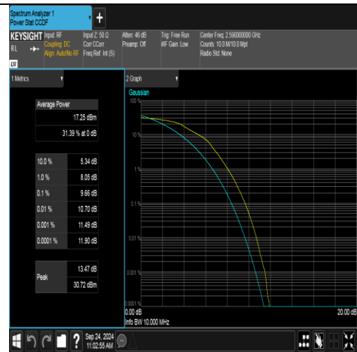
Band41(2535-2655)-10MHz-16QAM-40590-50RB#0-PASS
