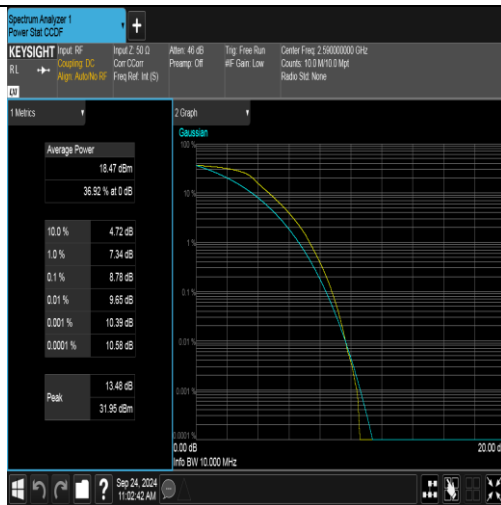
Band41(2535-2655)-10MHz-QPSK-40590-50RB#0-PASS
