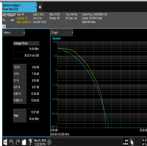
Band41(2535-2655)-20MHz-QPSK-41140-100RB#0-PASS
