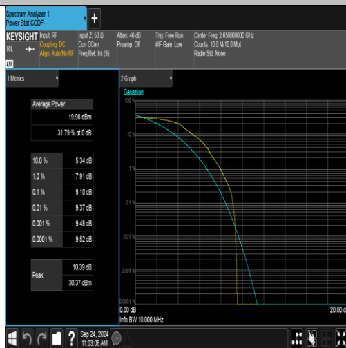
Band41(2535-2655)-10MHz-QPSK-41190-1RB#0-PASS
