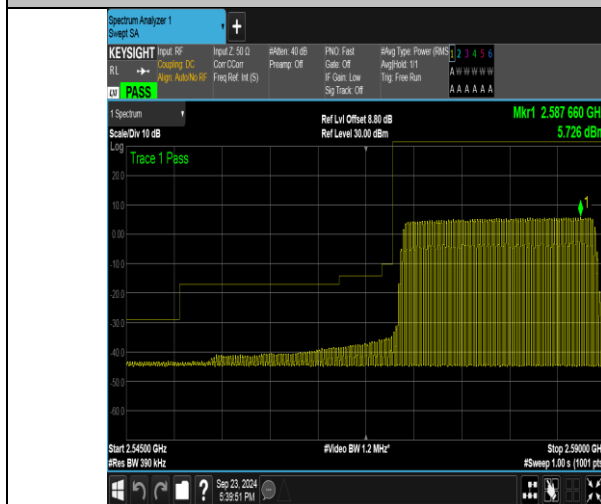
Band38_20MHz_QPSK_37850_100RB#0
