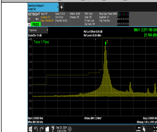
Band38_20MHz_QPSK_37850_1RB#0
