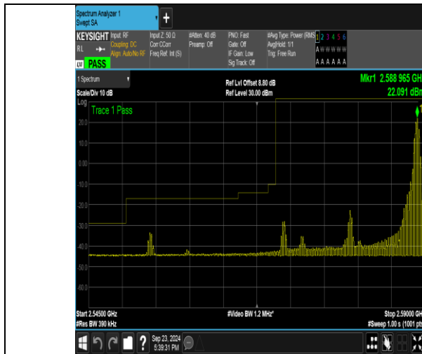
Band38_20MHz_QPSK_37850_1RB#99
