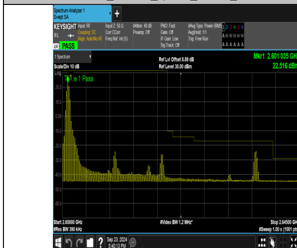
Band38_20MHz_QPSK_38150_1RB#0
