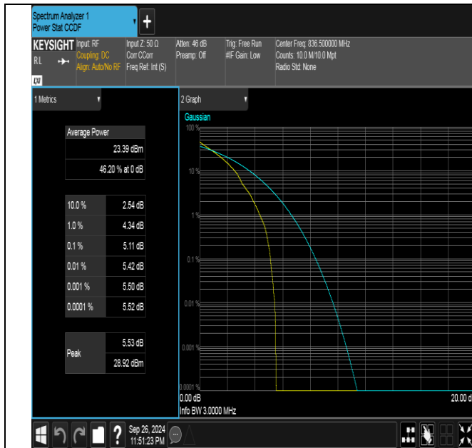
Band26(824-849)-3MHz-QPSK-26915-1RB#0-PASS
