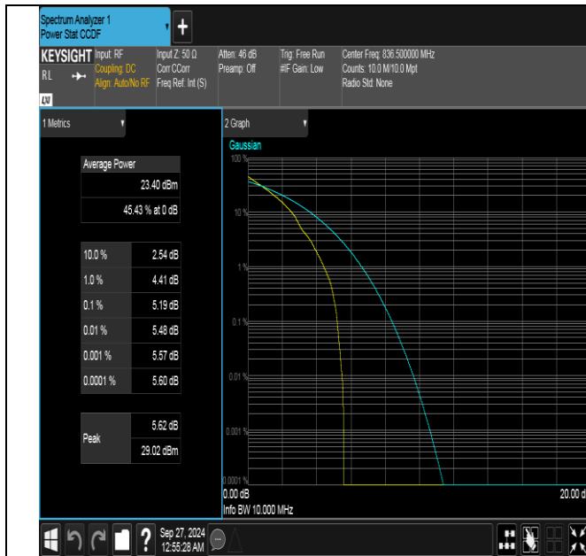
Band26(824-849)-10MHz-QPSK-26915-1RB#0-PASS
