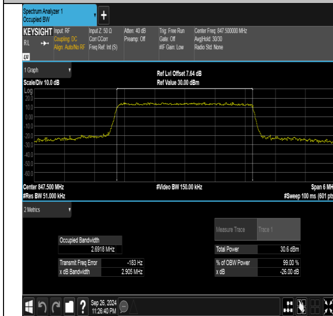
Band26(824-849)-3MHz-QPSK-27025-15RB#0-PASS
