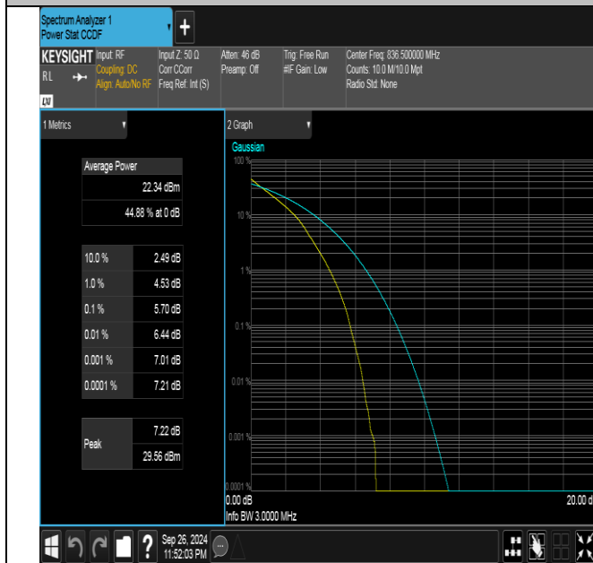
Band26(824-849)-3MHz-QPSK-26915-15RB#0-PASS
