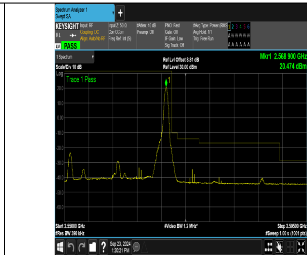
Band7_20MHz_16QAM_21350_1RB#99
