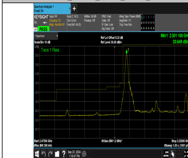
Band7_20MHz_QPSK_20850_1RB#0
