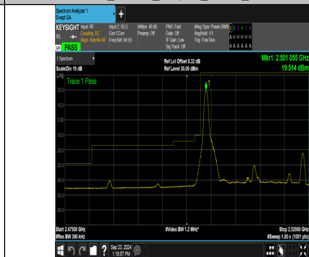
Band7_20MHz_16QAM_20850_1RB#0
