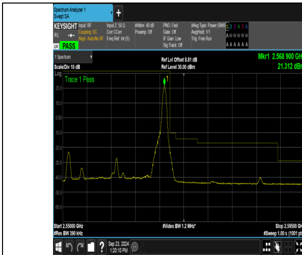
Band7_20MHz_QPSK_21350_1RB#99
