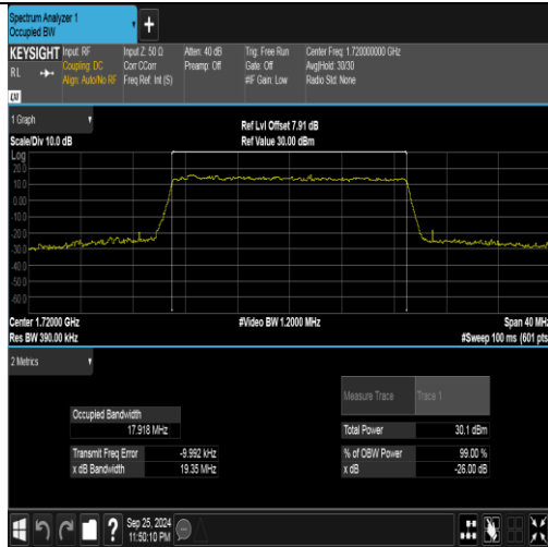
Band4-20MHz-QPSK-20050-100RB#0-PASS
