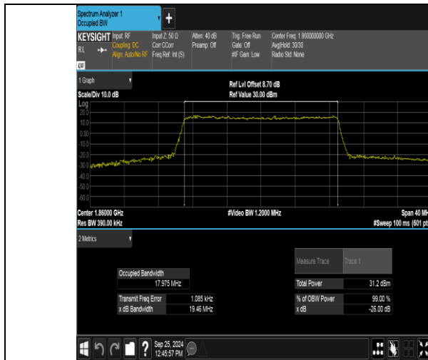
Band2-20MHz-QPSK-18700-100RB#0-PASS
