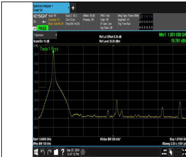
Band2_20MHz_QPSK_18700_1RB#0
