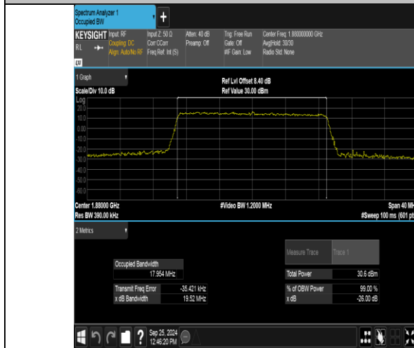
Band2-20MHz-QPSK-18900-100RB#0-PASS
