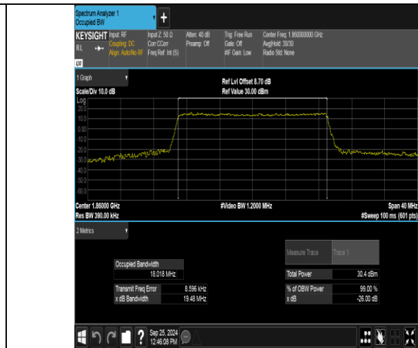
Band2-20MHz-16QAM-18700-100RB#0-PASS
