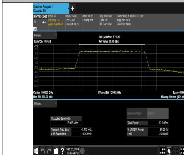
Band2-20MHz-QPSK-19100-100RB#0-PASS
