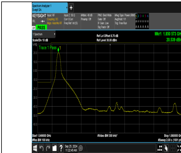
Band2_10MHz_QPSK_18650_1RB#0
