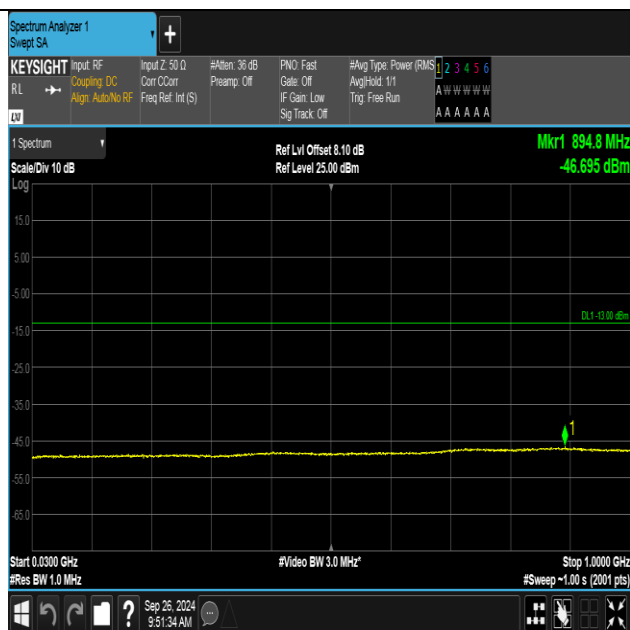
Band4-1312-4-30~1000MHz-PASS
