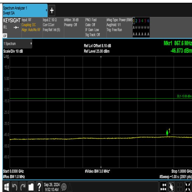
Band4-1413-4-30~1000MHz-PASS
