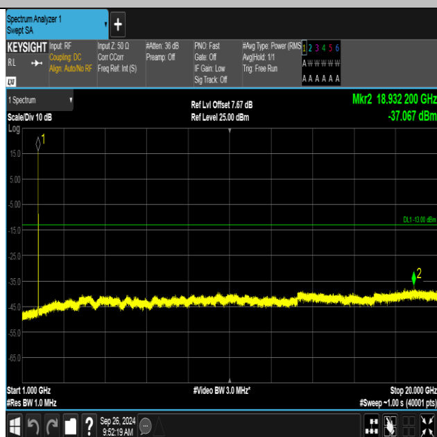
Band4-1413-4-1000~20000MHz-PASS
