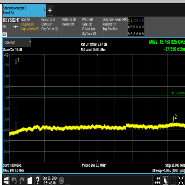
Band4-1312-4-1000~20000MHz-PASS
