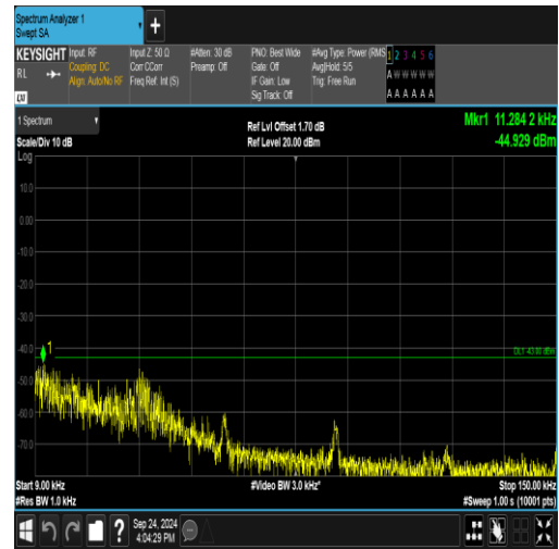
EGPRS1900-661-2-0.009~0.15MHz-PASS
