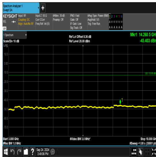
GPRS1900-661-0-3000~18000MHz-PASS
