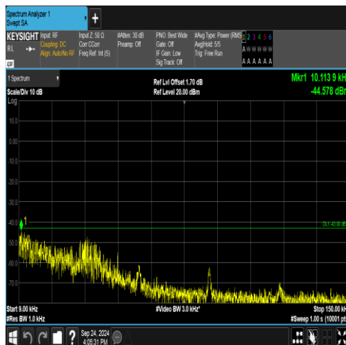
EGPRS1900-810-2-0.009~0.15MHz-PASS
