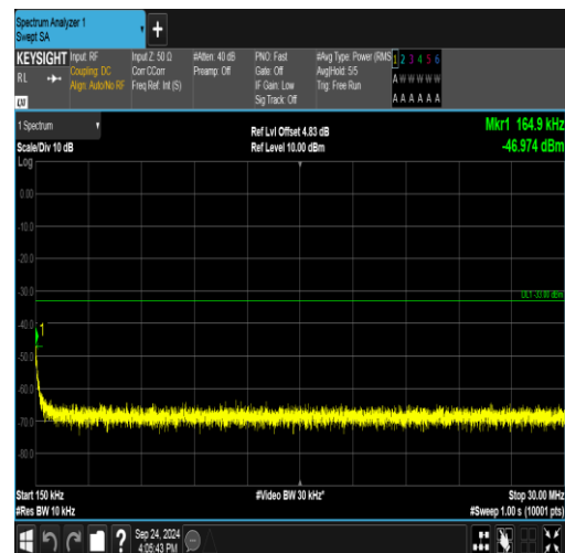
EGPRS1900-810-2-0.15~30MHz-PASS
