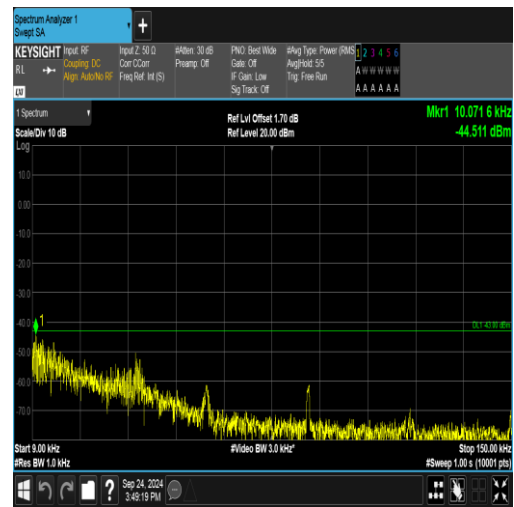
GPRS1900-810-0-0.009~0.15MHz-PASS
