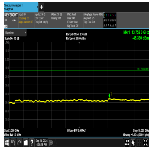
EGPRS1900-661-2-3000~18000MHz-PASS
