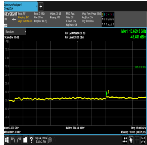
GSM1900-661-0-3000~18000MHz-PASS
