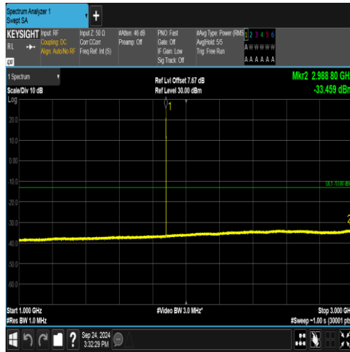
GSM1900-661-0-1000~3000MHz-PASS
