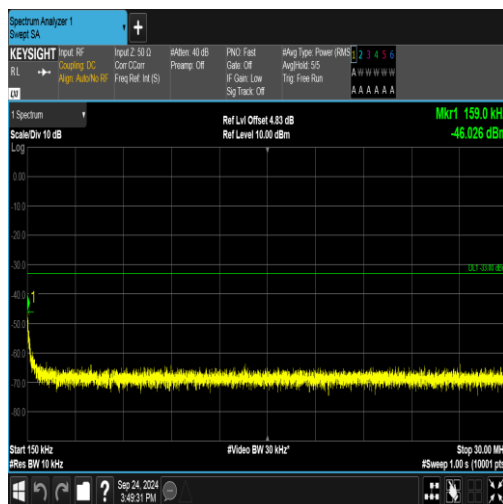
GPRS1900-810-0-0.15~30MHz-PASS
