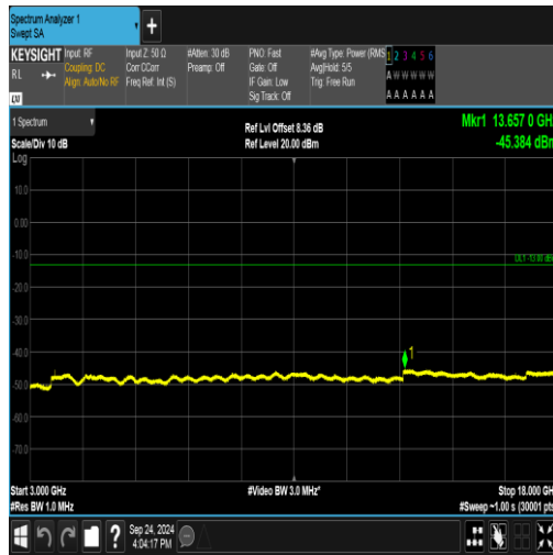
EGPRS1900-512-2-3000~18000MHz-PASS
