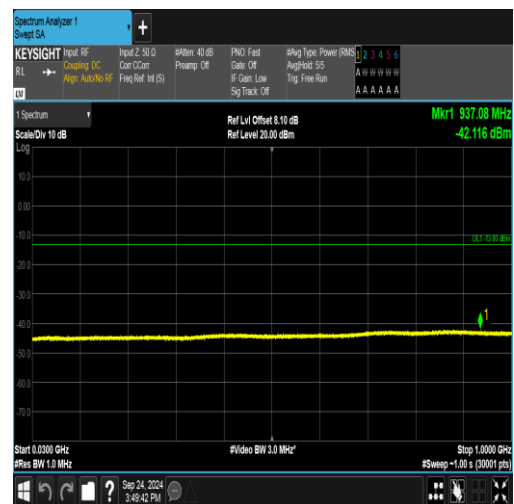
GPRS1900-810-0-30~1000MHz-PASS
