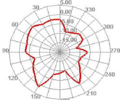
2450.000MHz E1
