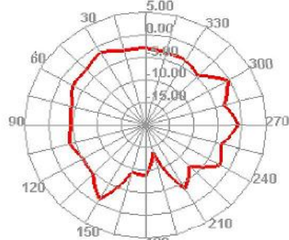
2450.000MHz E2
