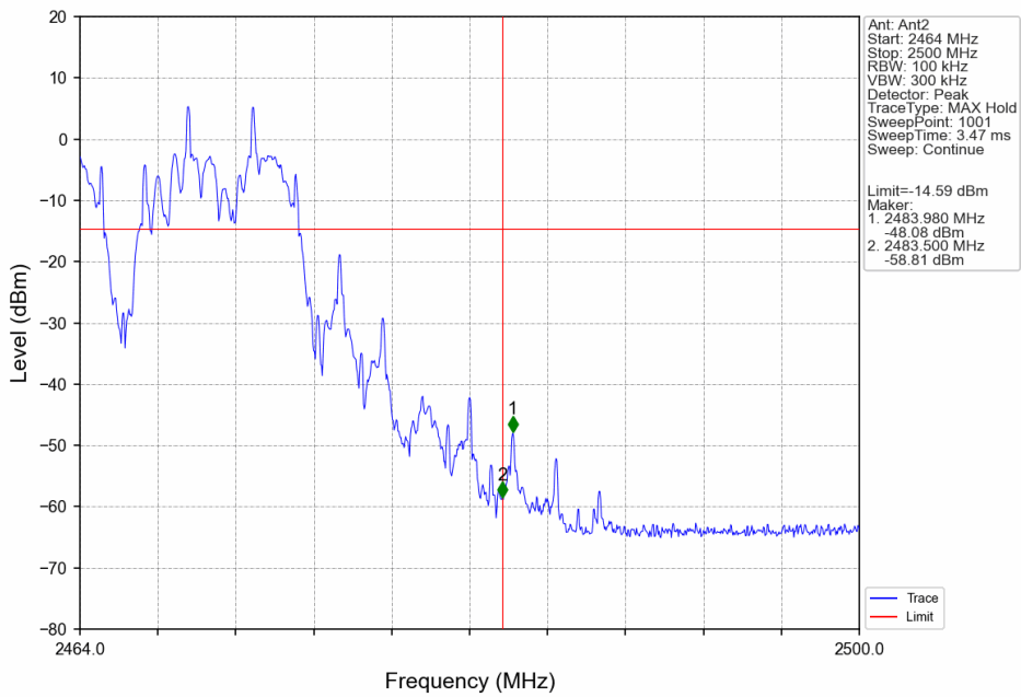
GFSK_HOPP_Ant2_NTNV
