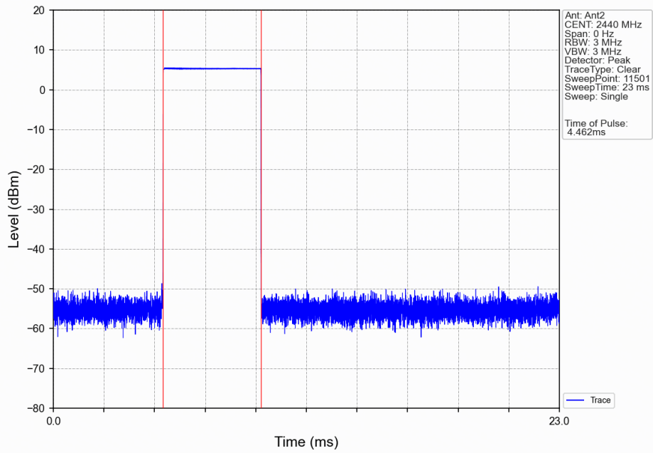
GFSK_HOPP_Ant2_NTNV
