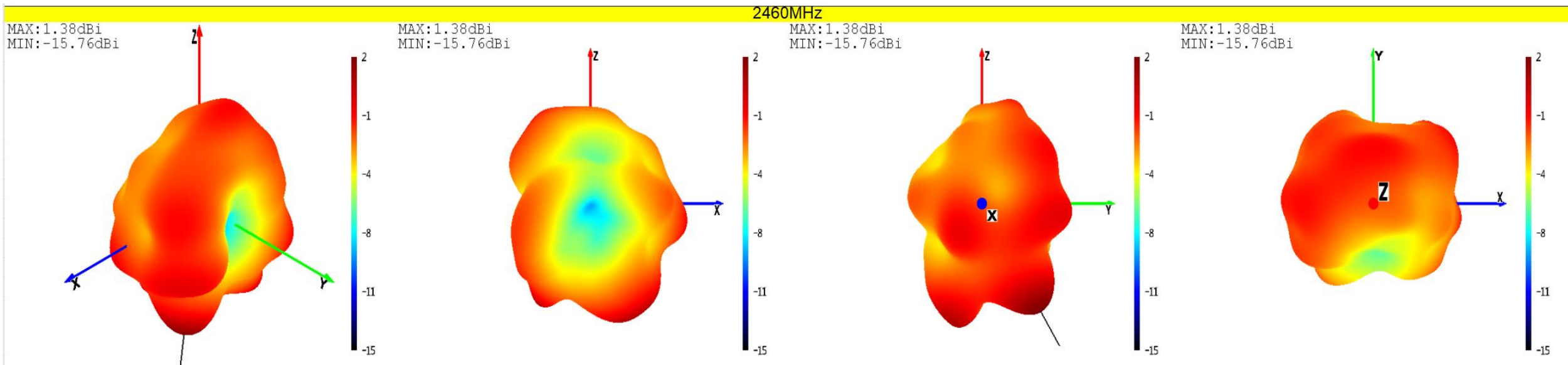
Theta=0 Freq=2460MHz
