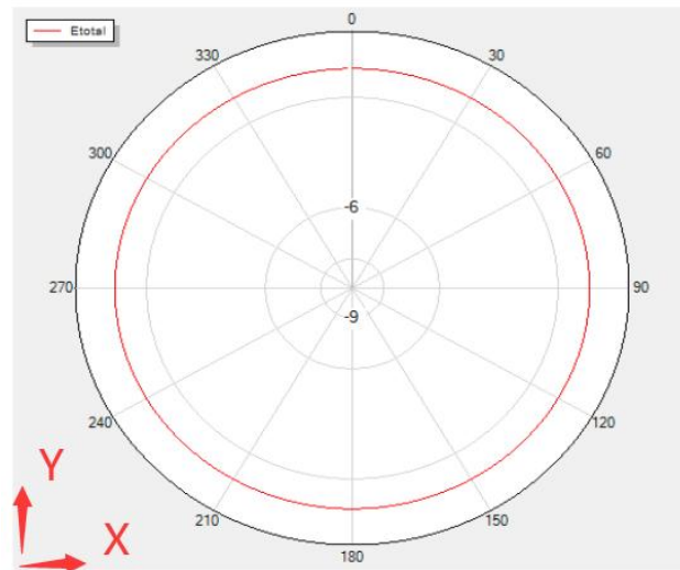
Theta=0 Freq=2460MHz
