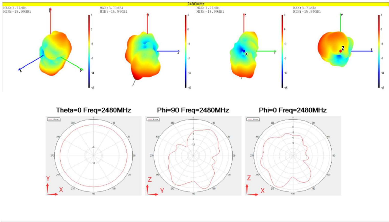
2480MHz天线苹果图和方向图
