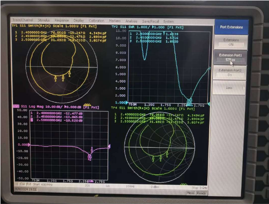
天线smith圆图和S11参数
