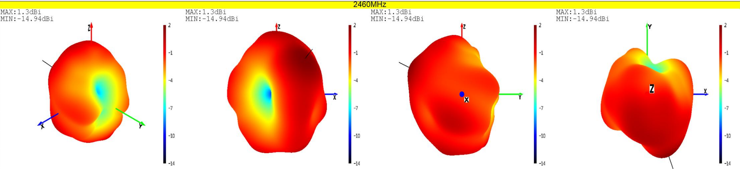
Theta=0 Freq=2460MHz
