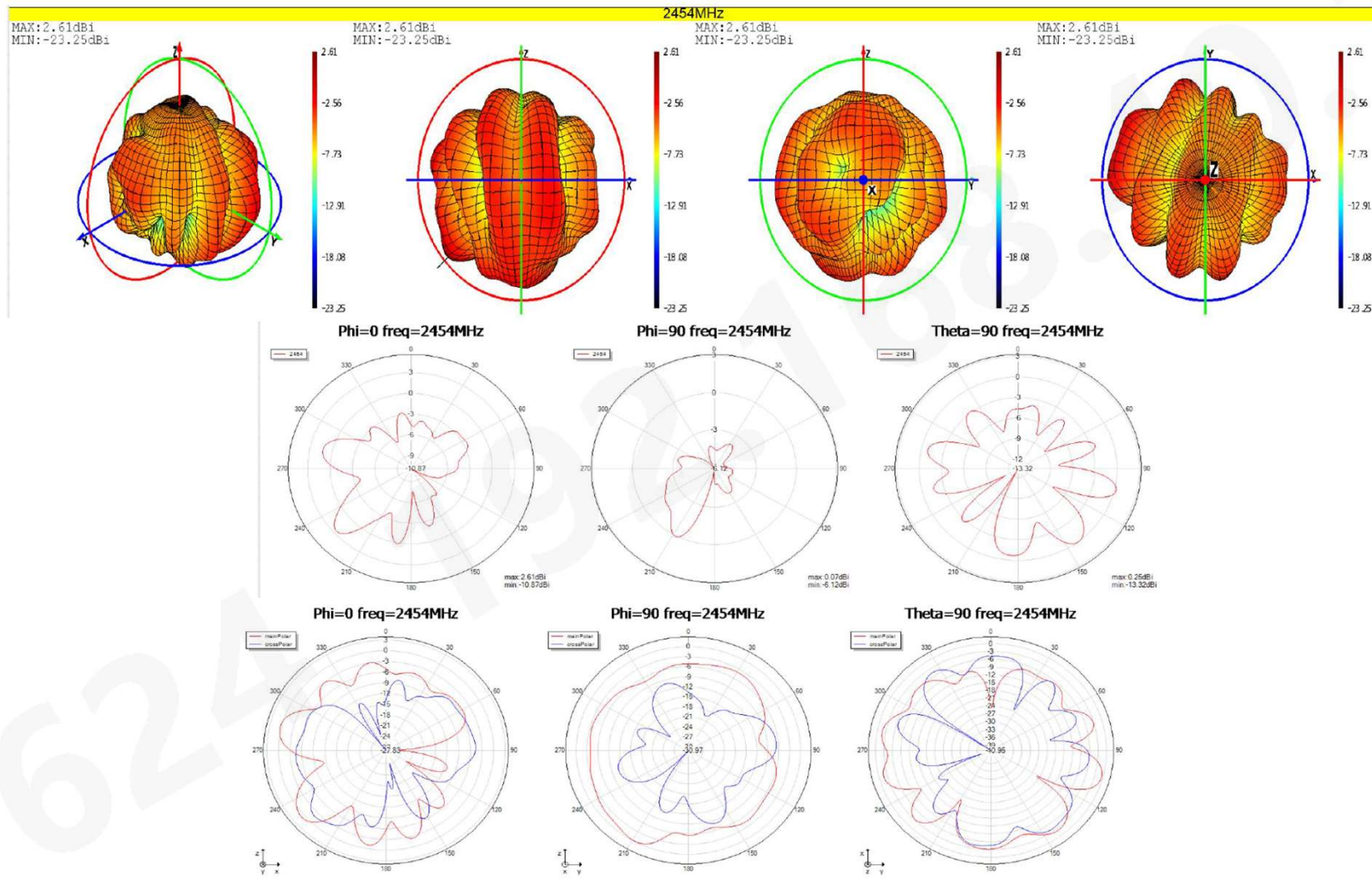
天线苹果图和方向图
