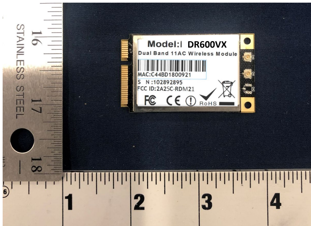
Front of 5 GHz Mini PCIe Radio Module (Radios 1 & 2)
