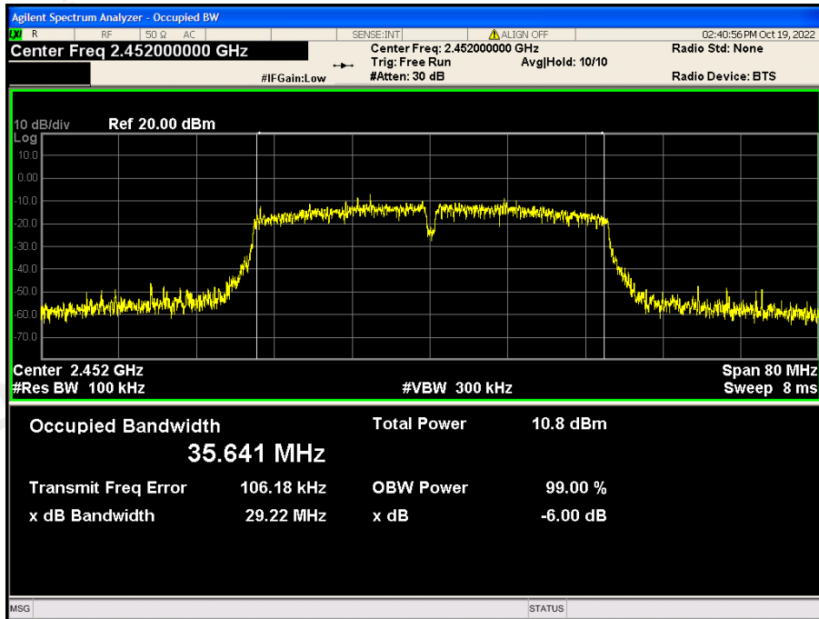
CH09: 2452MHz
