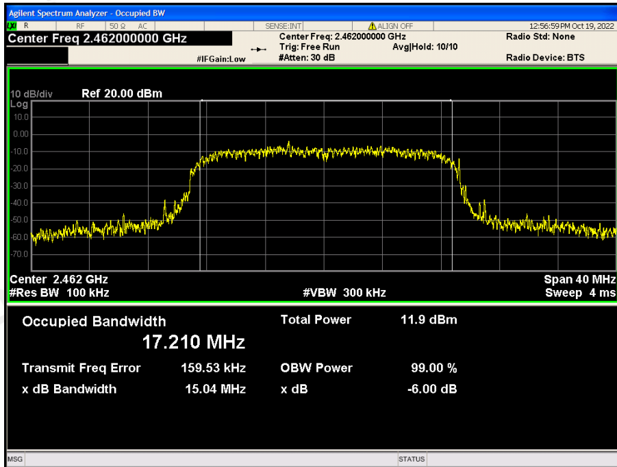
CH11: 2462MHz
