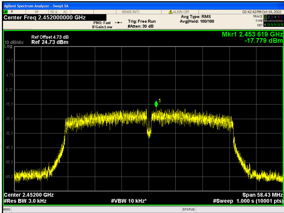
CH09: 2452MHz
