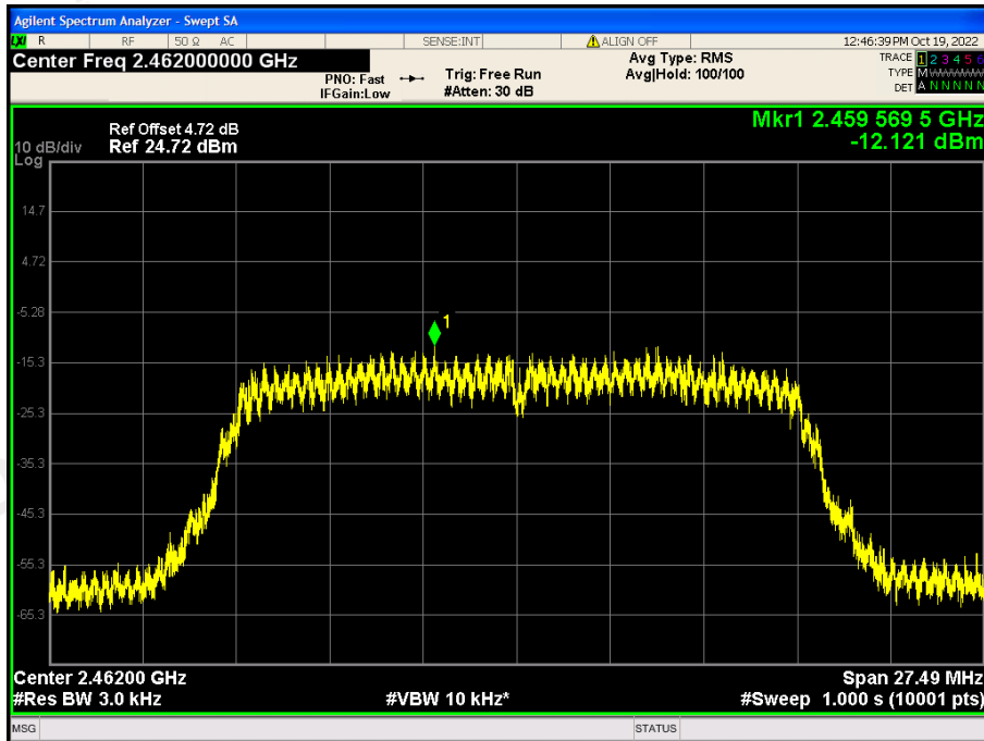
CH11: 2462MHz
