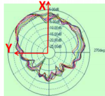
E2 (Phi=90)
