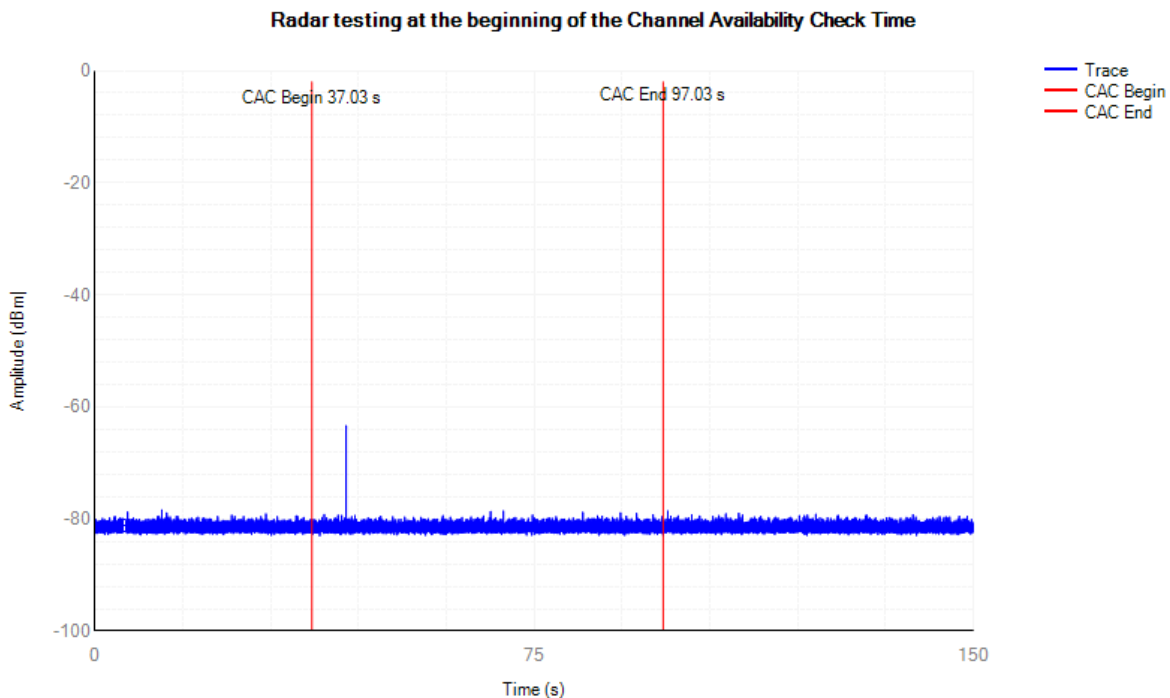
802.11ax HE80 5530MHz
