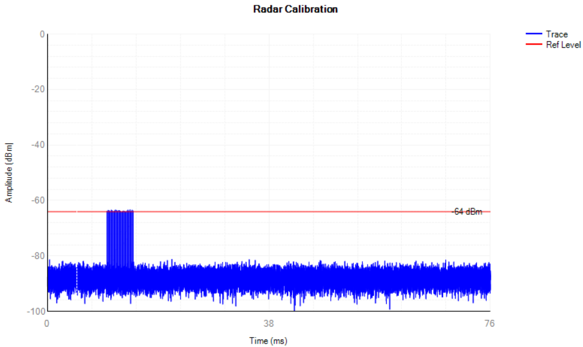
802.11ax HE20 5500MHz_Type3
