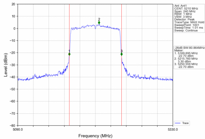
802.11ac(VHT80) MCH_5290MHz_AntA_NTNV
