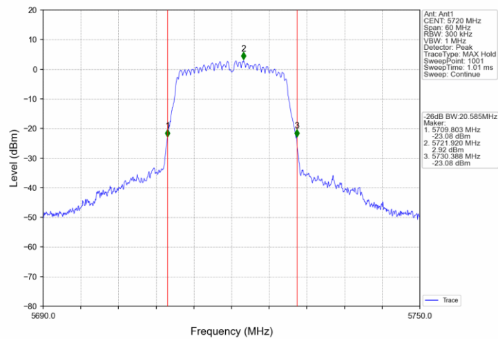
802.11n(HT40)_LCH_5190MHz_AntA_NTNV
