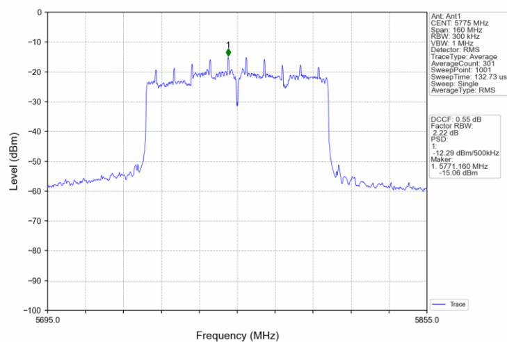
802.11ac(VHT80) MCH_5775MHz_AntA_NTNV
