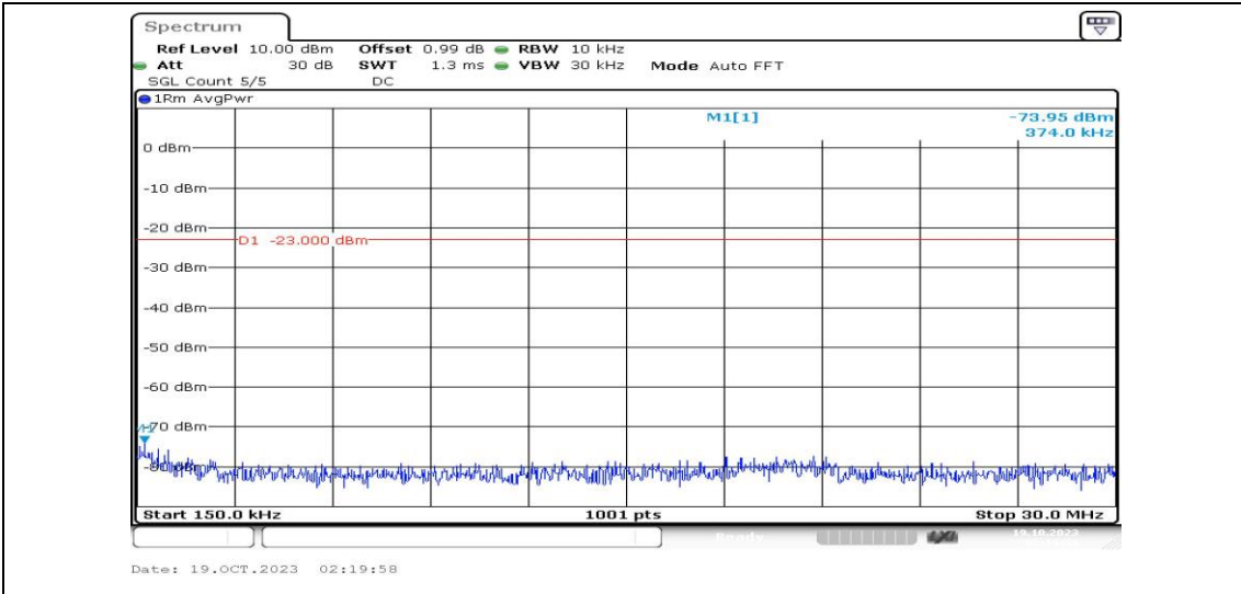
Band5-10MHz-QPSK-20525-1RB#0-Range2:0.15~30MHz-PASS
