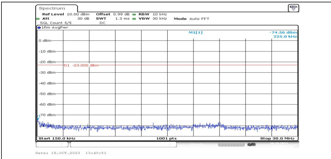
Band5-3MHz-QPSK-20635-1RB#0-Range2:0.15~30MHz-PASS
