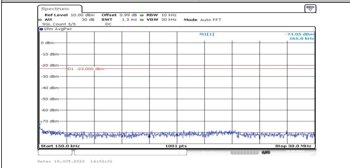
Band5-5MHz-QPSK-20425-1RB#0-Range2:0.15~30MHz-PASS
