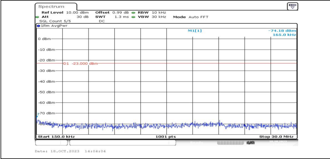
Band5-5MHz-QPSK-20525-1RB#0-Range2:0.15~30MHz-PASS
