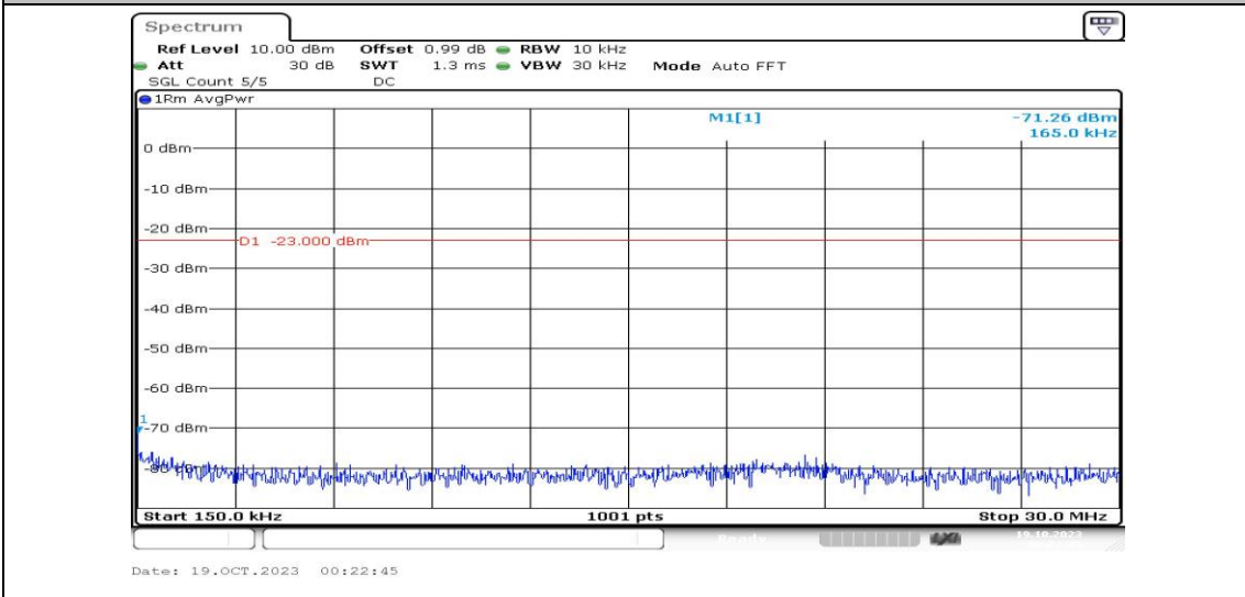
Band4-20MHz-QPSK-20050-1RB#0-Range2:0.15~30MHz-PASS
