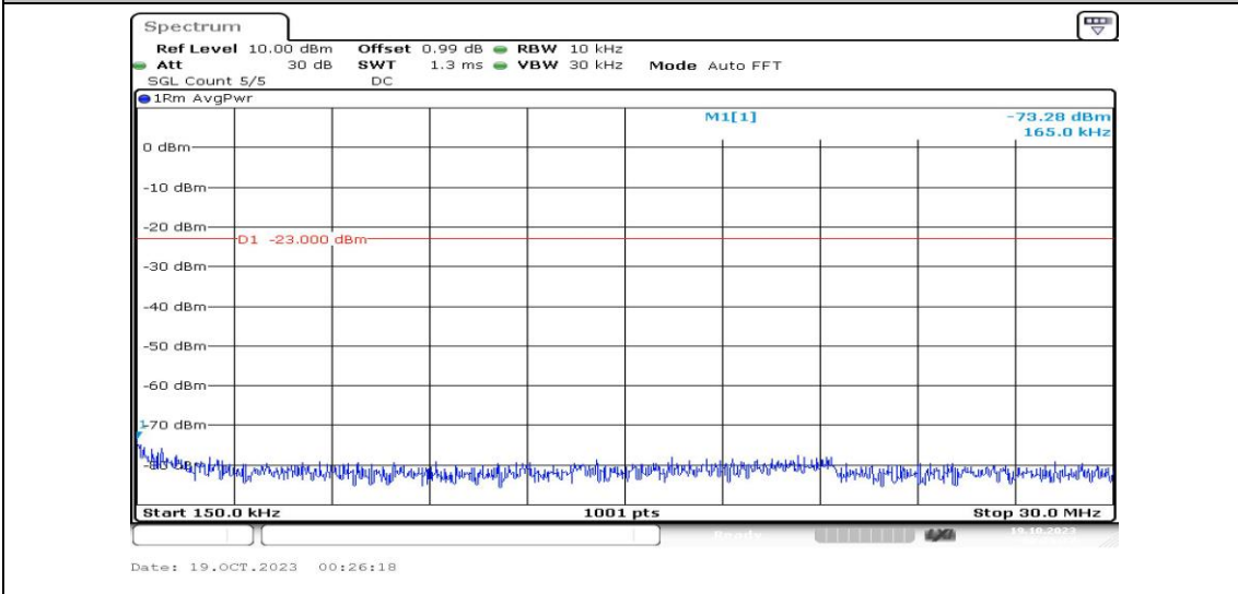
Band4-20MHz-QPSK-20300-1RB#0-Range2:0.15~30MHz-PASS
