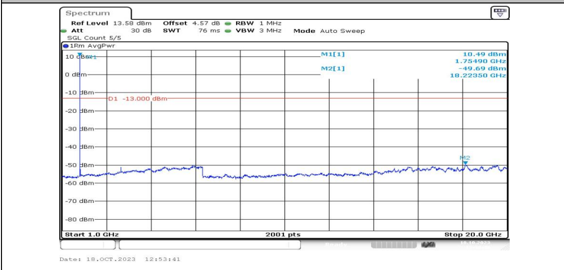
Band4-5MHz-QPSK-20375-1RB#0-Range4:1000~20000MHz-PASS
