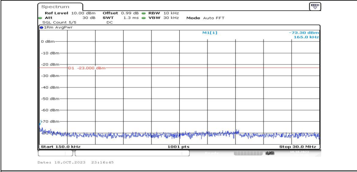
Band4-10MHz-QPSK-20000-1RB#0-Range2:0.15~30MHz-PASS
