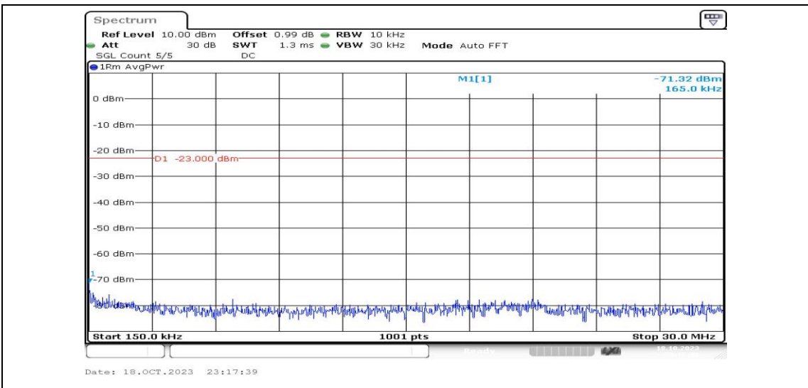
Band4-10MHz-QPSK-20175-1RB#0-Range2:0.15~30MHz-PASS
