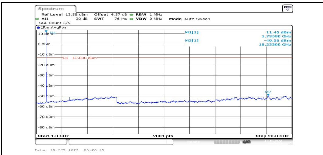
Band4-20MHz-QPSK-20300-1RB#0-Range4:1000~20000MHz-PASS
