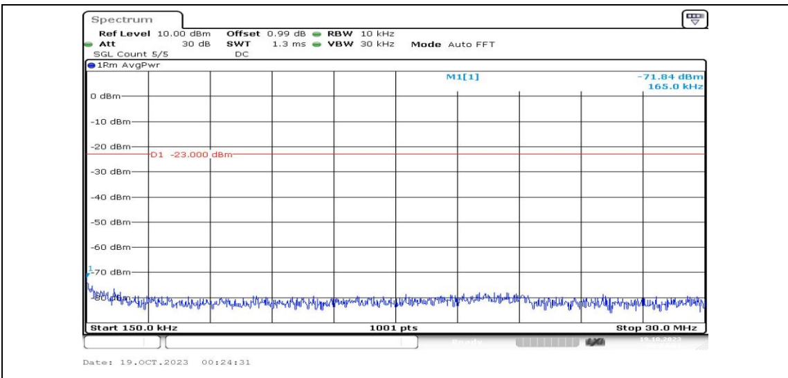
Band4-20MHz-QPSK-20175-1RB#0-Range2:0.15~30MHz-PASS
