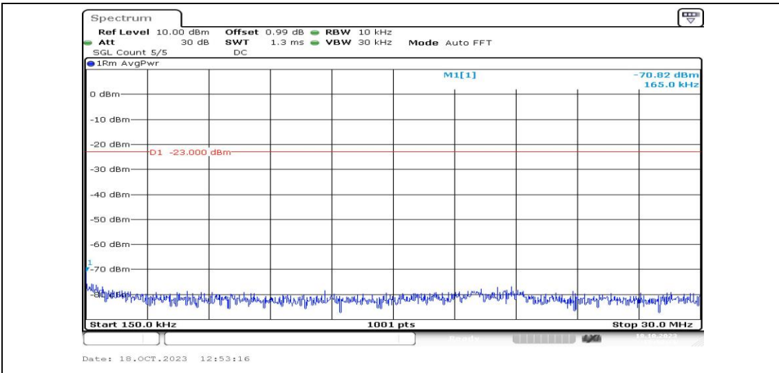
Band4-5MHz-QPSK-20375-1RB#0-Range2:0.15~30MHz-PASS
