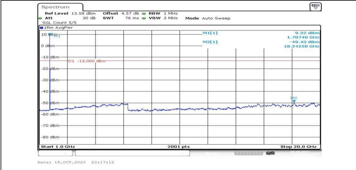
Band4-10MHz-QPSK-20000-1RB#0-Range4:1000~20000MHz-PASS
