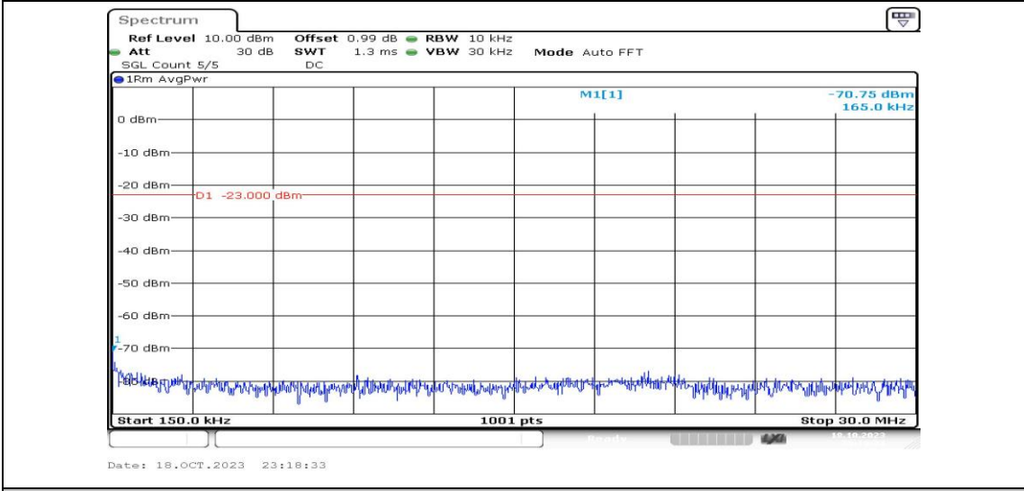
Band4-10MHz-QPSK-20350-1RB#0-Range2:0.15~30MHz-PASS
