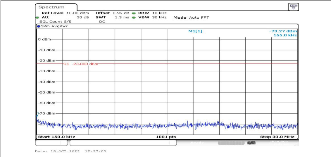
Band4-3MHz-QPSK-20175-1RB#0-Range2:0.15~30MHz-PASS
