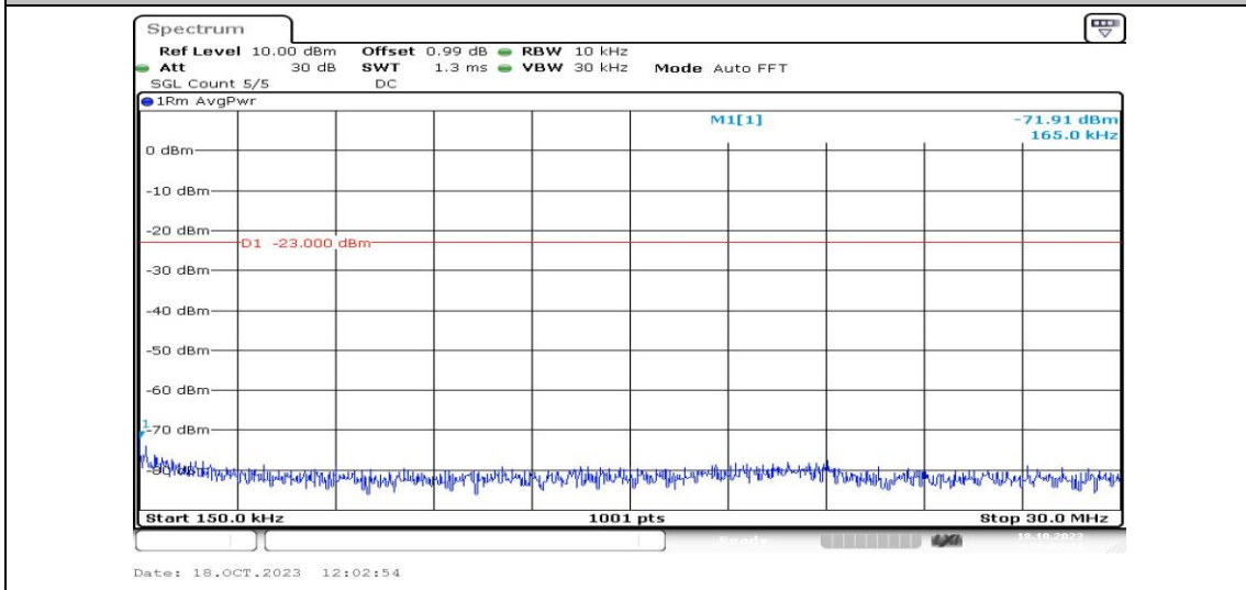
Band4-1.4MHz-QPSK-20175-1RB#0-Range2:0.15~30MHz-PASS
