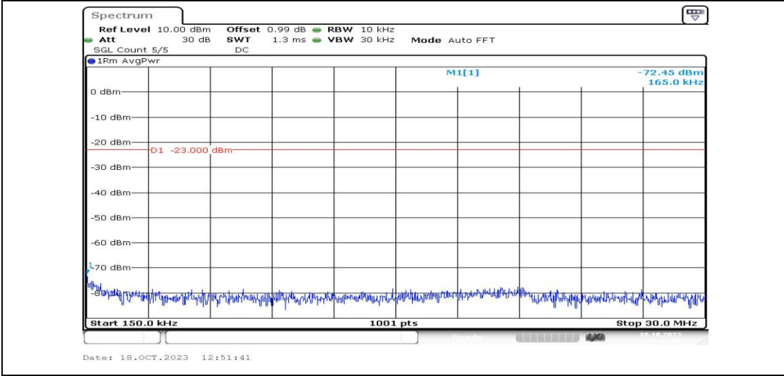
Band4-5MHz-QPSK-20175-1RB#0-Range2:0.15~30MHz-PASS
