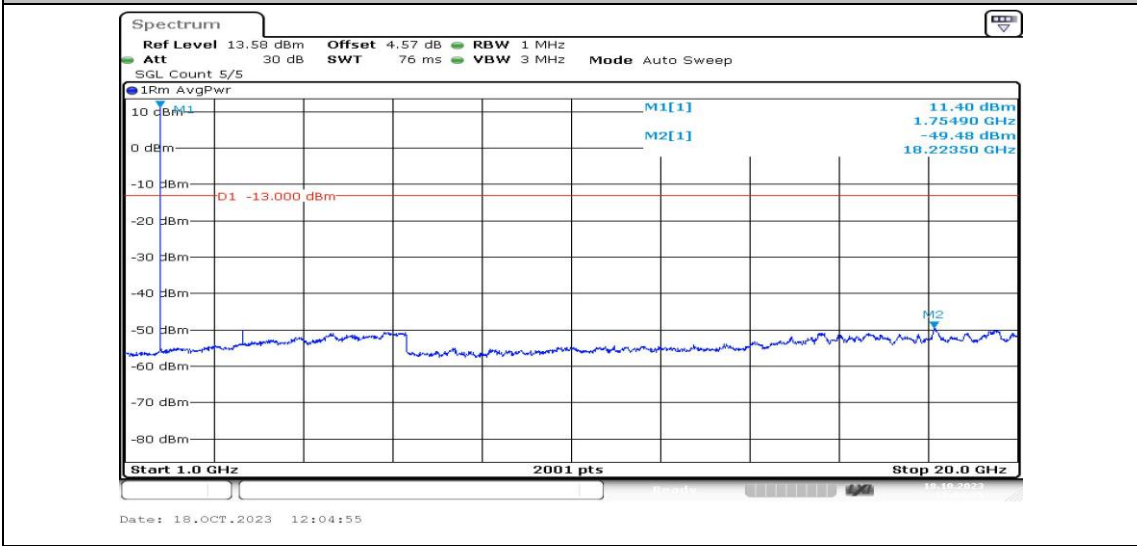
Band4-1.4MHz-QPSK-20393-1RB#0-Range4:1000~20000MHz-PASS
