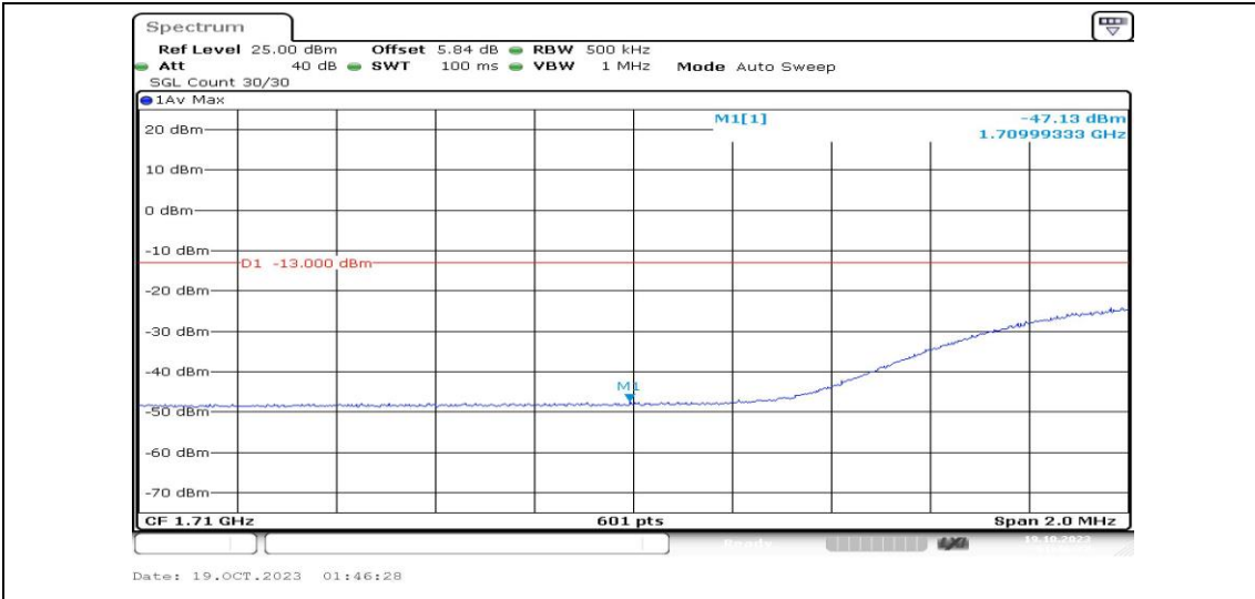
Band4-20MHz-16QAM-20050-1RB#99-PASS
