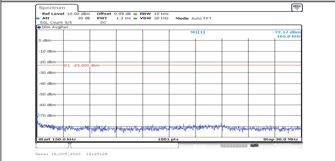
Band4-3MHz-QPSK-19965-1RB#0-Range2:0.15~30MHz-PASS
