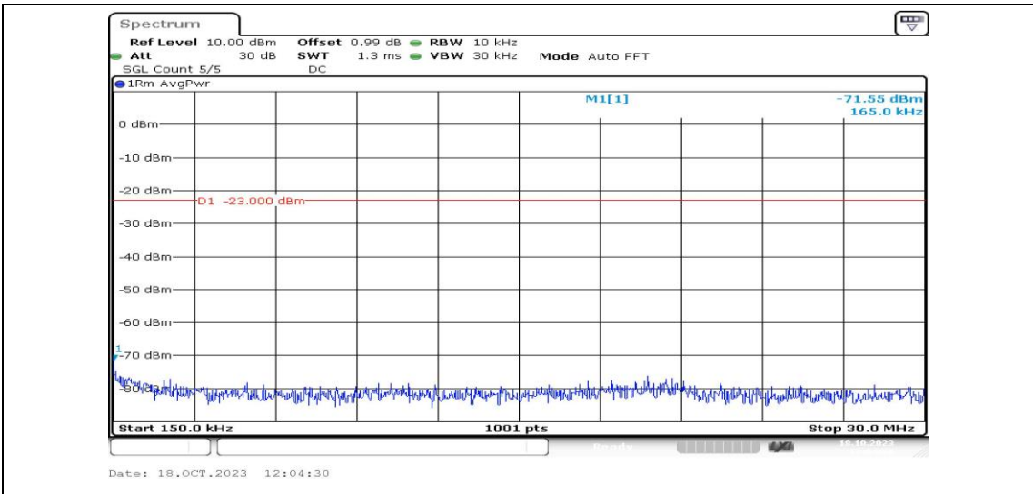
Band4-1.4MHz-QPSK-20393-1RB#0-Range2:0.15~30MHz-PASS
