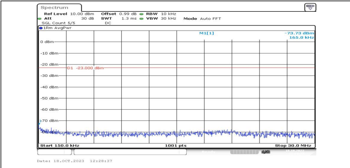
Band4-3MHz-QPSK-20385-1RB#0-Range2:0.15~30MHz-PASS
