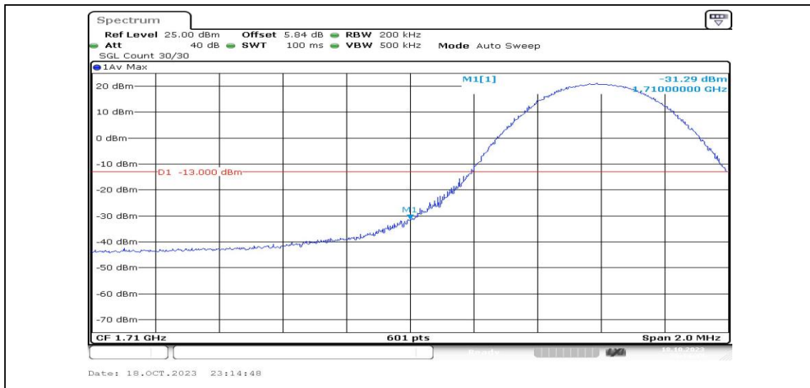
Band4-10MHz-QPSK-20000-1RB#0-PASS
