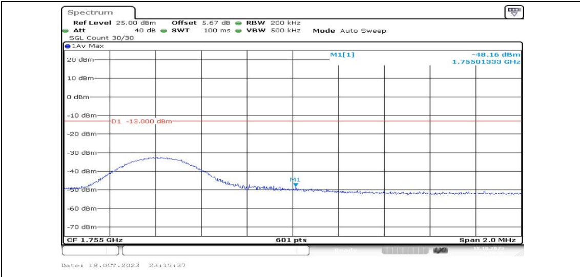
Band4-10MHz-QPSK-20350-1RB#0-PASS
