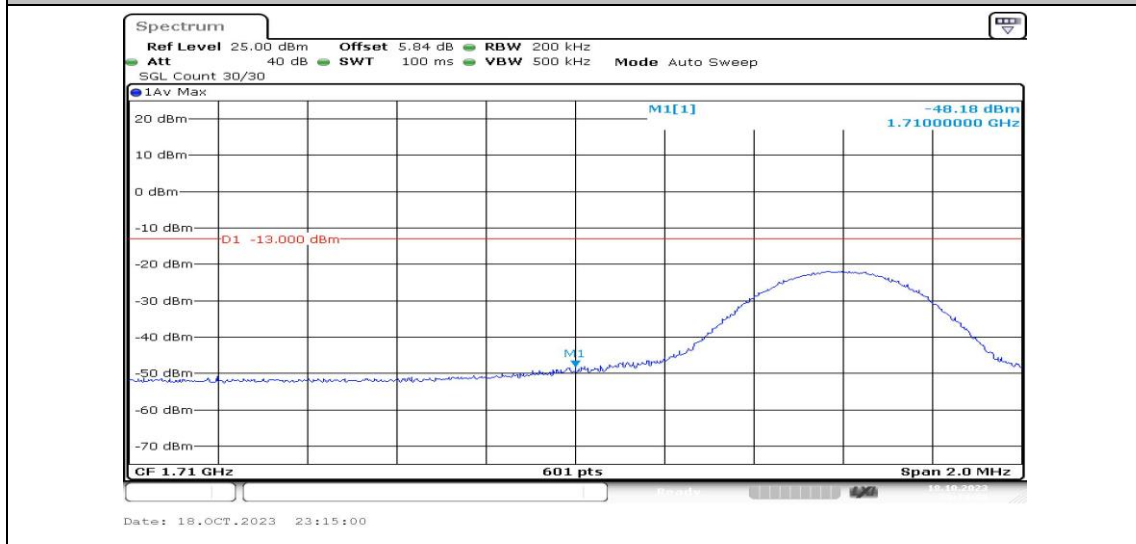
Band4-10MHz-QPSK-20000-1RB#49-PASS
