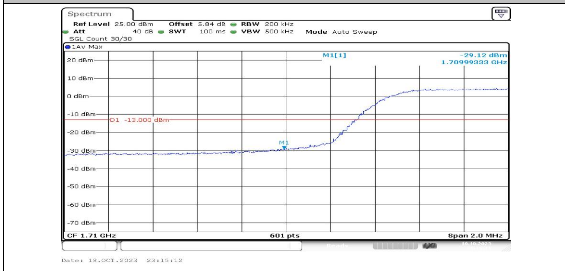
Band4-10MHz-QPSK-20000-50RB#0-PASS
