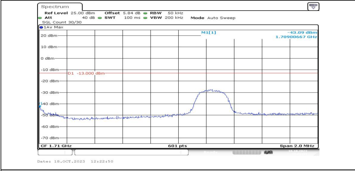
Band4-3MHz-QPSK-19965-1RB#14-PASS
