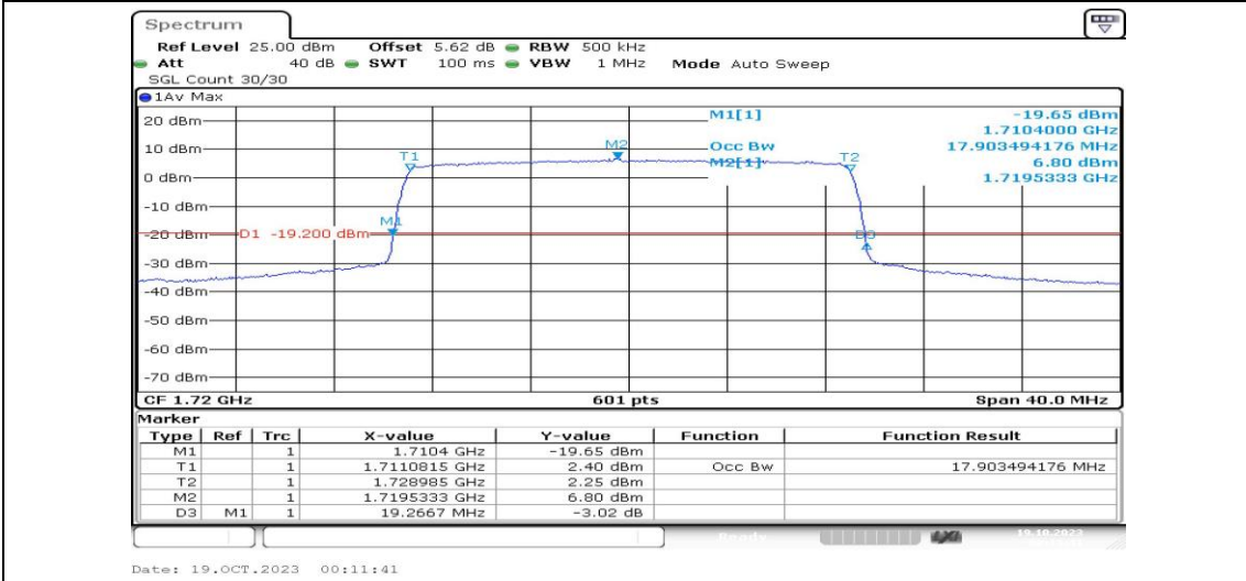
Band4-20MHz-QPSK-20050-100RB#0-PASS
