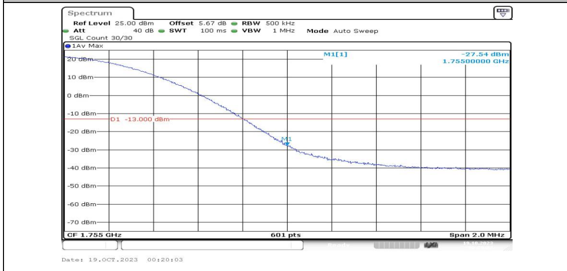
Band4-20MHz-QPSK-20300-1RB#99-PASS
