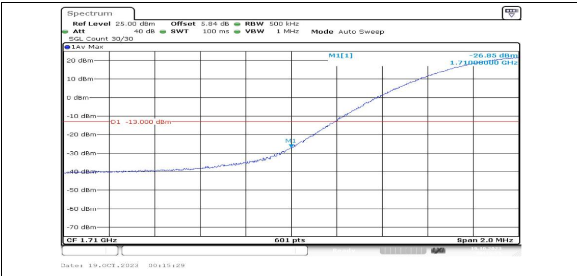
Band4-20MHz-QPSK-20050-1RB#0-PASS
