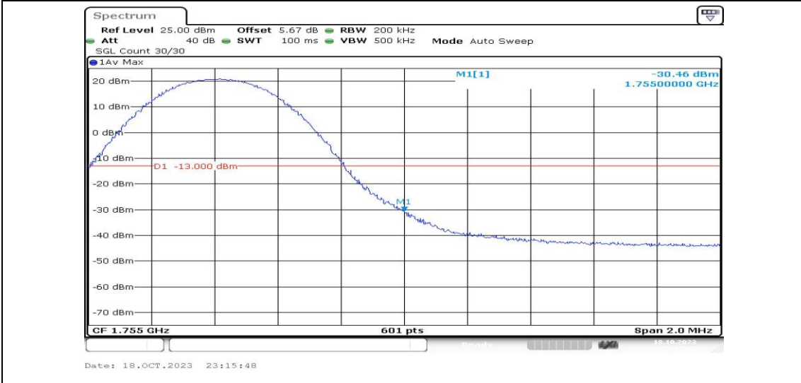
Band4-10MHz-QPSK-20350-1RB#49-PASS
