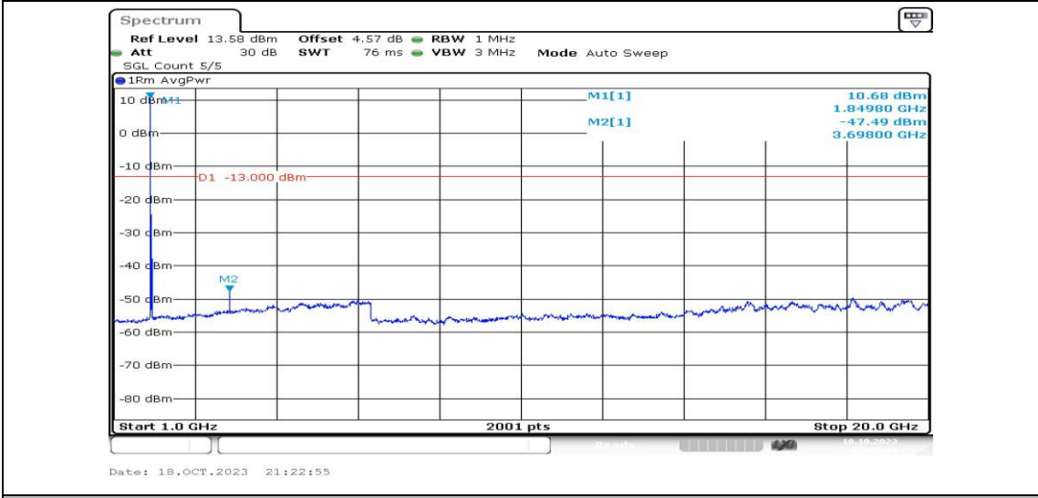
Band2-20MHz-QPSK-18700-1RB#0-Range4:1000~20000MHz-PASS
