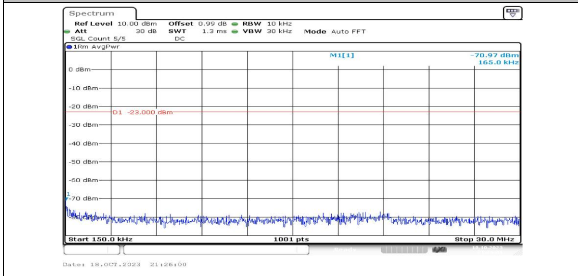
Band2-20MHz-QPSK-19100-1RB#0-Range2:0.15~30MHz-PASS
