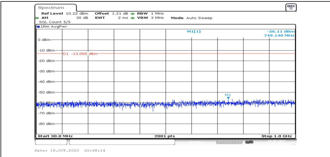
Band2-20MHz-16QAM-18700-1RB#0-Range3:30~1000MHz-PASS
