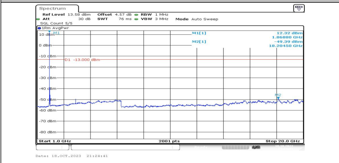
Band2-20MHz-QPSK-18900-1RB#0-Range4:1000~20000MHz-PASS
