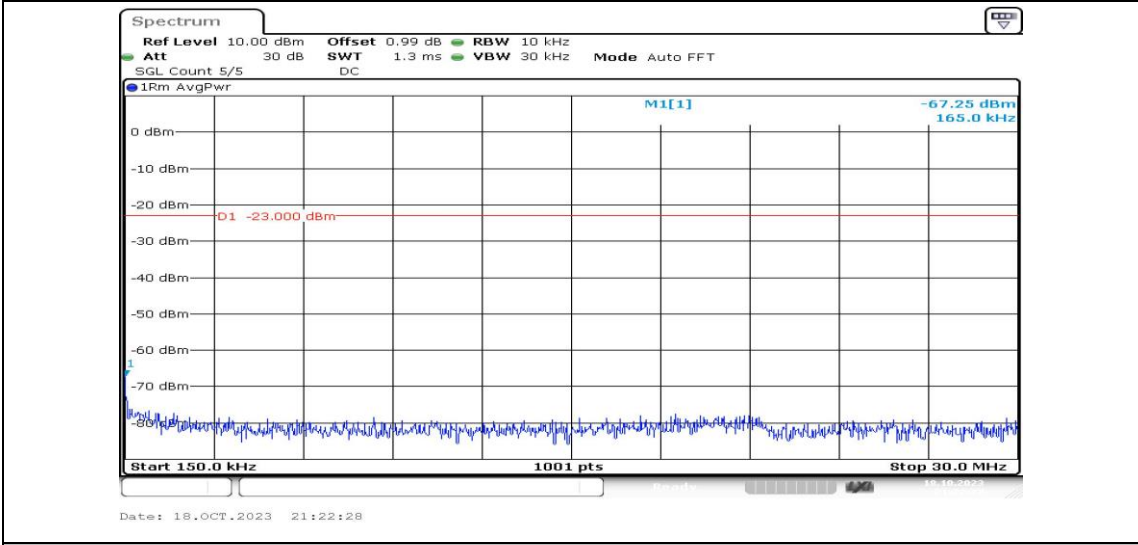
Band2-20MHz-QPSK-18700-1RB#0-Range2:0.15~30MHz-PASS
