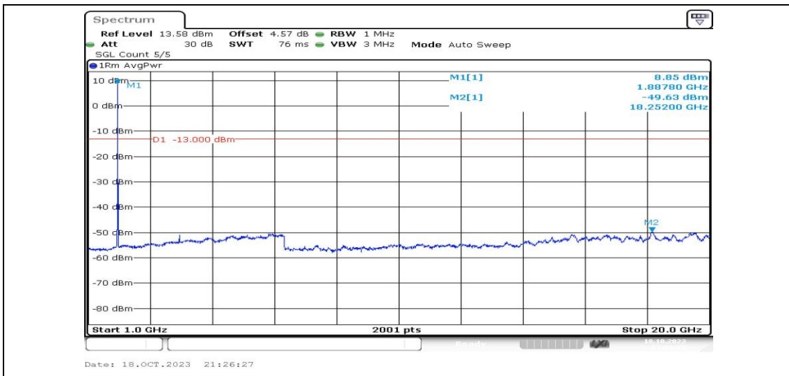
Band2-20MHz-QPSK-19100-1RB#0-Range4:1000~20000MHz-PASS
