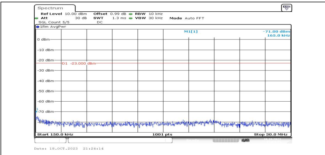
Band2-20MHz-QPSK-18900-1RB#0-Range2:0.15~30MHz-PASS
