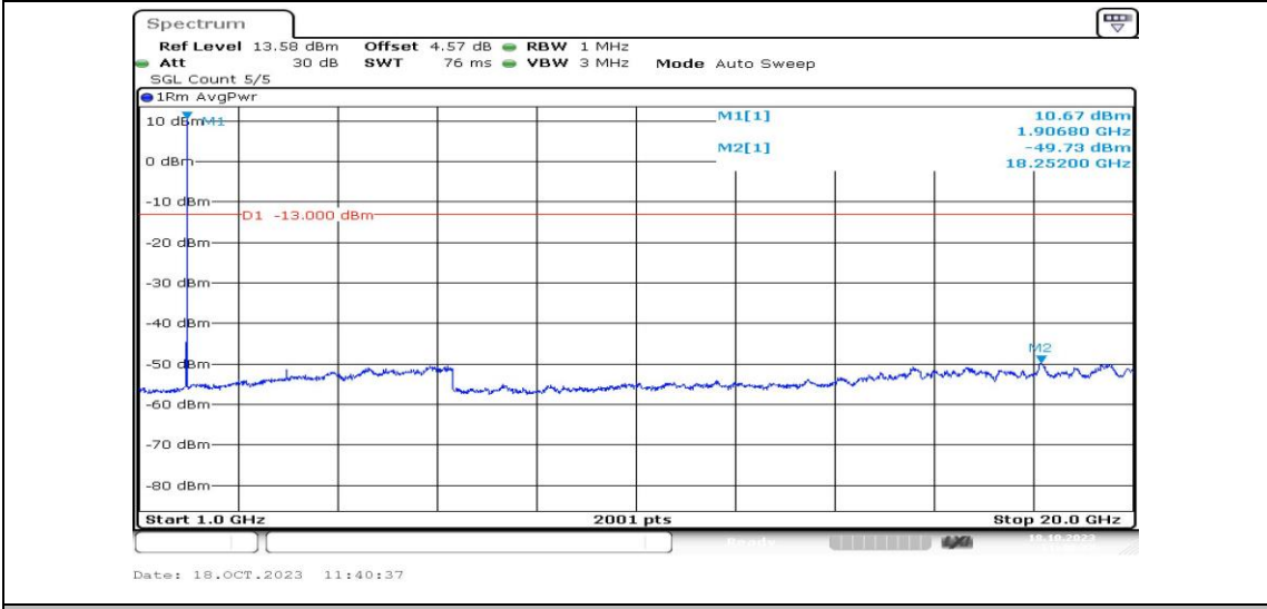
Band2-5MHz-QPSK-19175-1RB#0-Range4:1000~20000MHz-PASS
