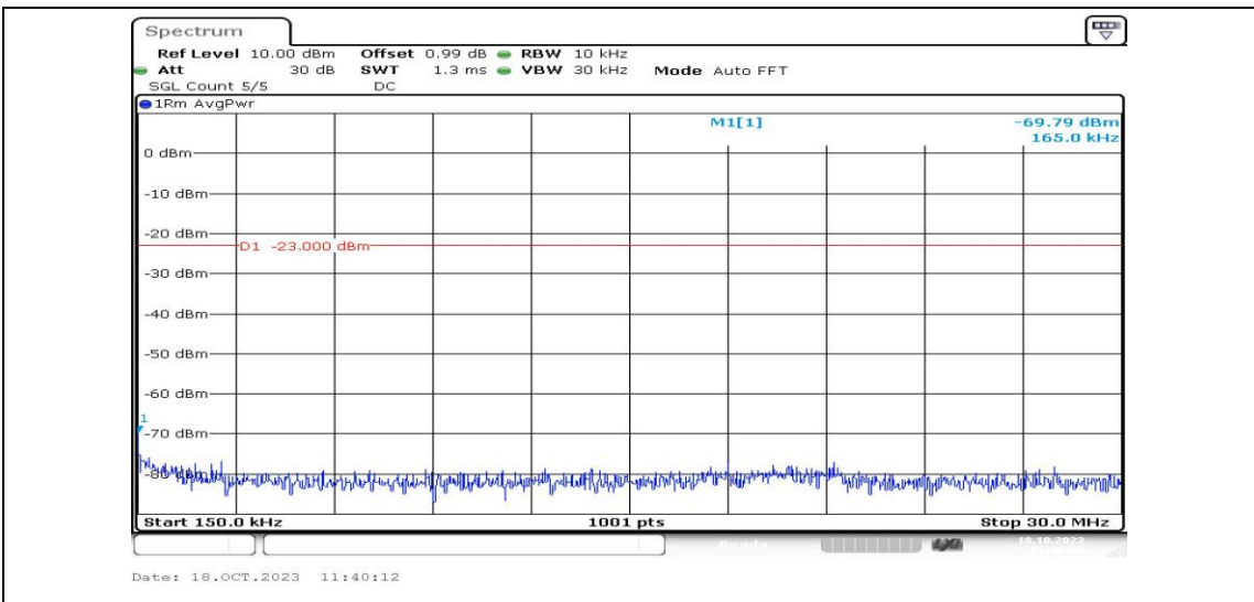
Band2-5MHz-QPSK-19175-1RB#0-Range2:0.15~30MHz-PASS
