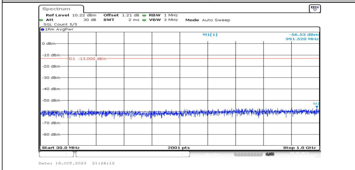
Band2-20MHz-QPSK-19100-1RB#0-Range3:30~1000MHz-PASS
