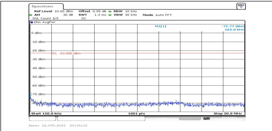
Band2-10MHz-QPSK-18900-1RB#0-Range2:0.15~30MHz-PASS
