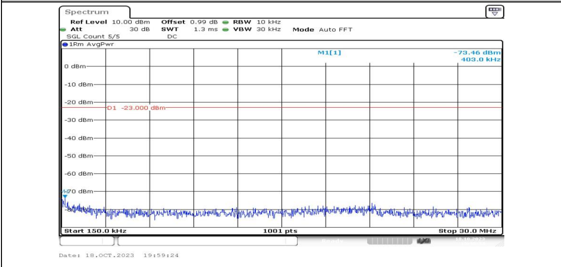
Band2-10MHz-QPSK-18650-1RB#0-Range2:0.15~30MHz-PASS
