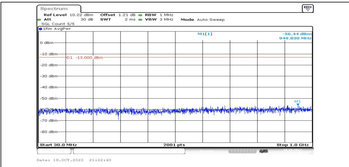
Band2-20MHz-QPSK-18700-1RB#0-Range3:30~1000MHz-PASS
