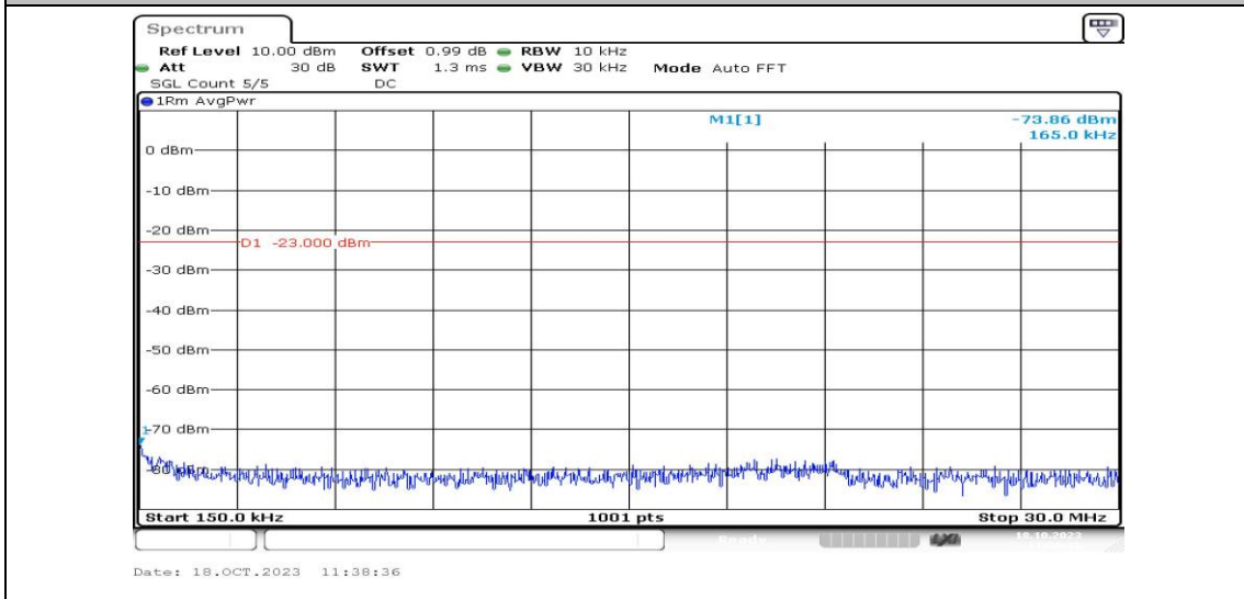
Band2-5MHz-QPSK-18900-1RB#0-Range2:0.15~30MHz-PASS
