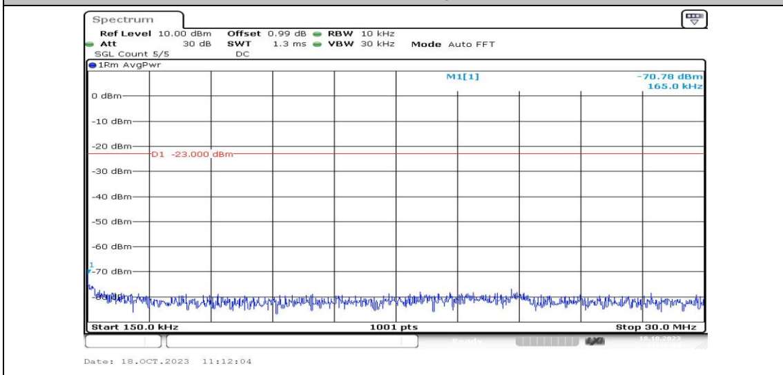
Band2-3MHz-QPSK-18615-1RB#0-Range2:0.15~30MHz-PASS
