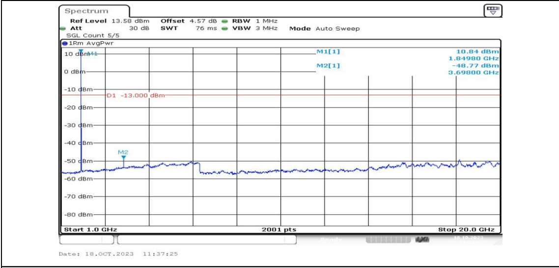
Band2-5MHz-QPSK-18625-1RB#0-Range4:1000~20000MHz-PASS
