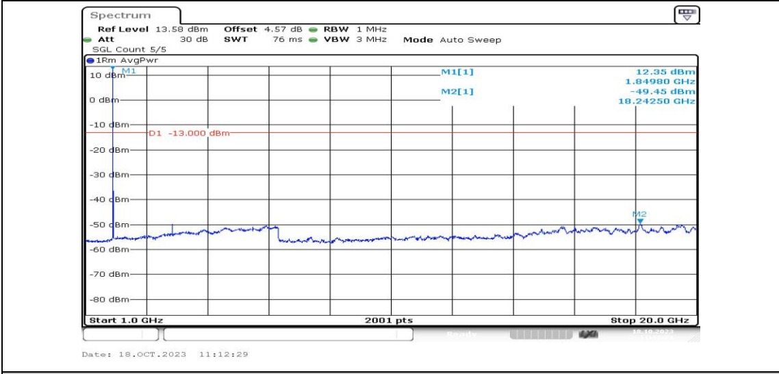
Band2-3MHz-QPSK-18615-1RB#0-Range4:1000~20000MHz-PASS
