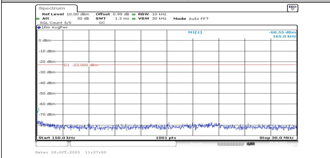
Band2-5MHz-QPSK-18625-1RB#0-Range2:0.15~30MHz-PASS
