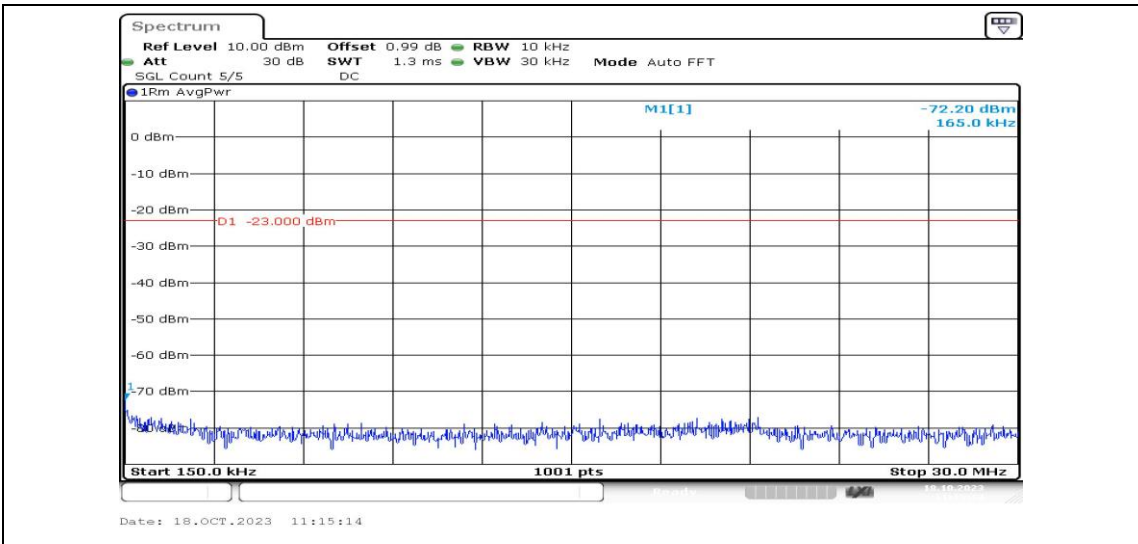
Band2-3MHz-QPSK-19185-1RB#0-Range2:0.15~30MHz-PASS
