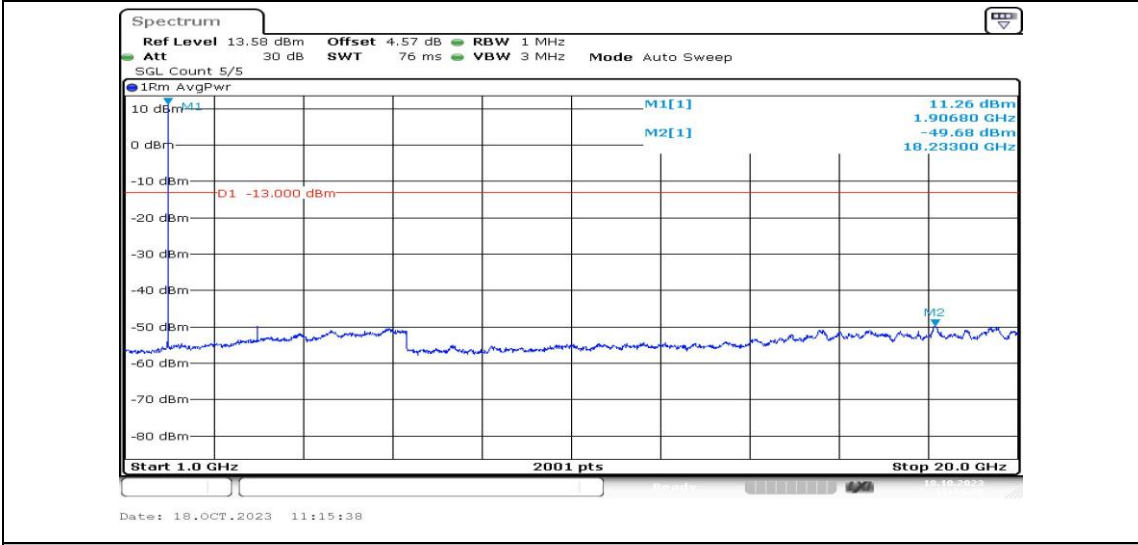
Band2-3MHz-QPSK-19185-1RB#0-Range4:1000~20000MHz-PASS
