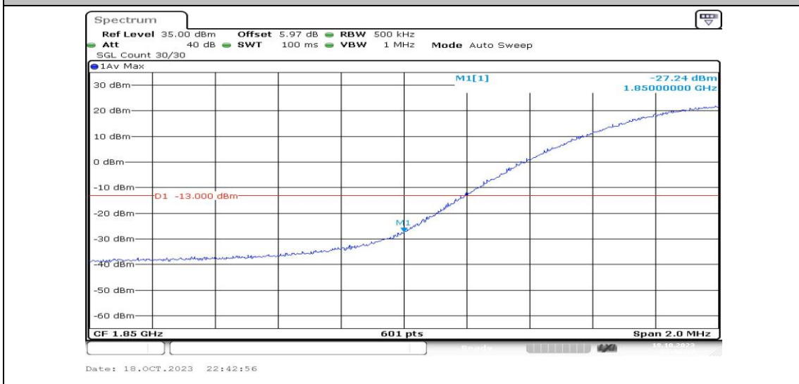
Band2-20MHz-16QAM-18700-1RB#0-PASS
