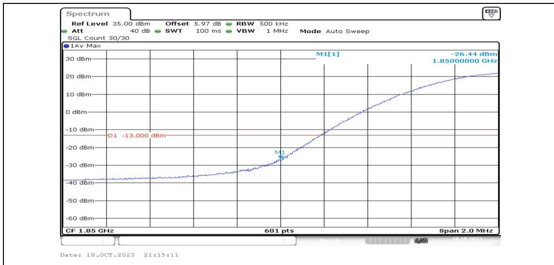
Band2-20MHz-QPSK-18700-1RB#0-PASS
