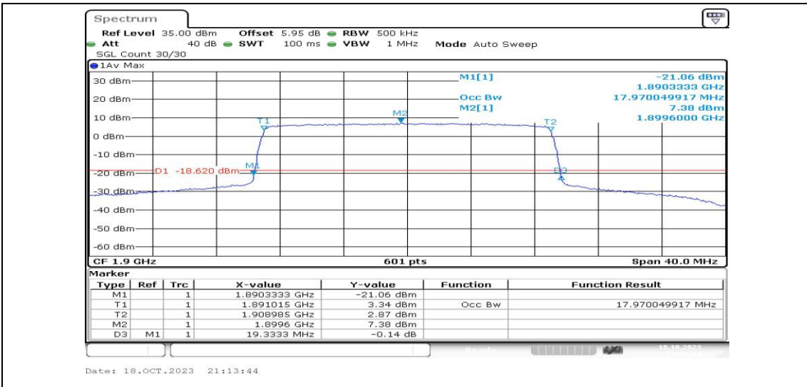
Band2-20MHz-QPSK-19100-100RB#0-PASS
