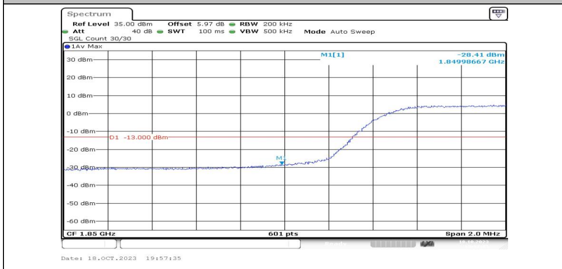
Band2-10MHz-QPSK-18650-50RB#0-PASS
