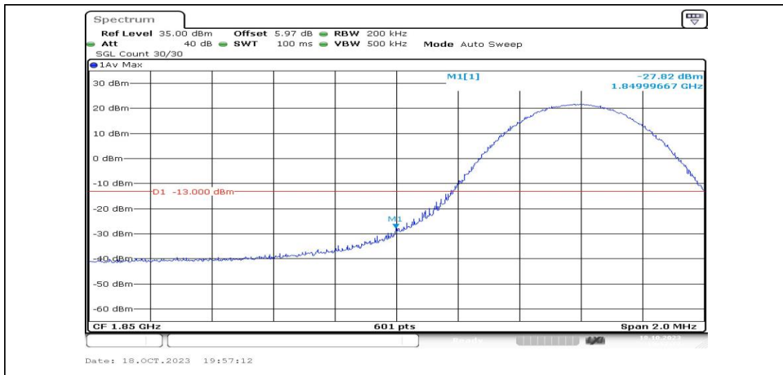
Band2-10MHz-QPSK-18650-1RB#0-PASS
