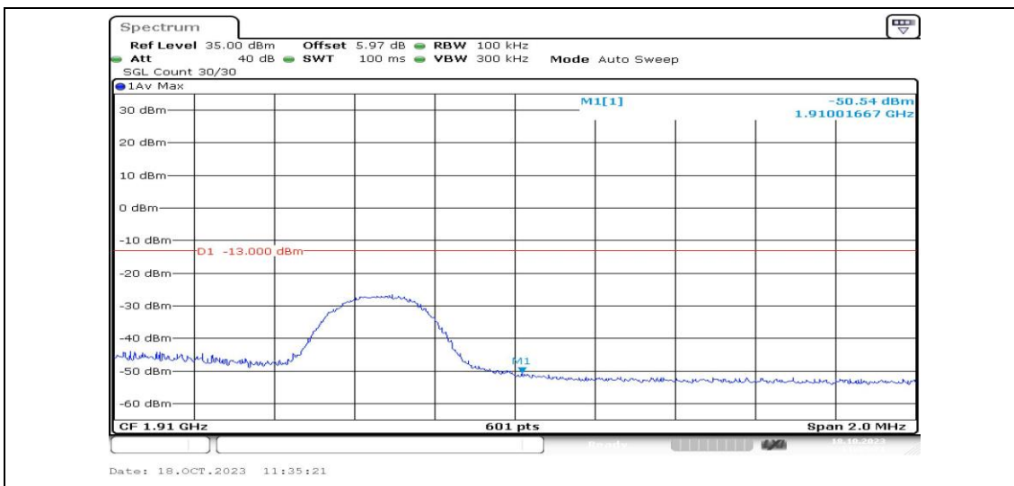
Band2-5MHz-QPSK-19175-1RB#0-PASS
