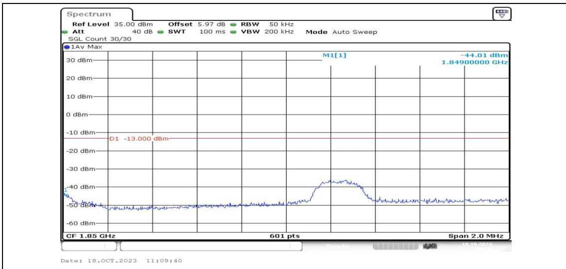
Band2-3MHz-16QAM-18615-1RB#14-PASS
