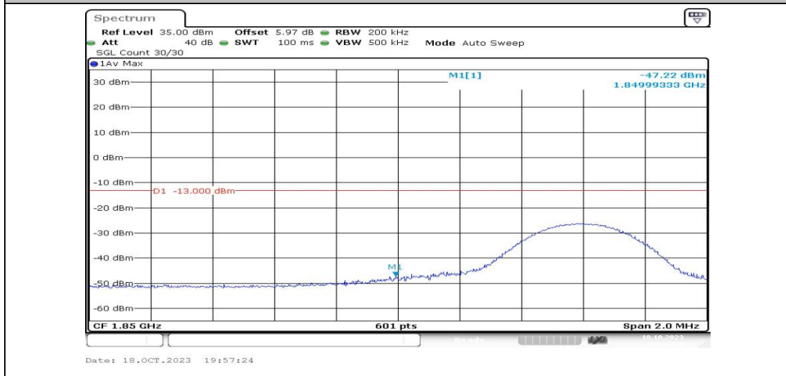
Band2-10MHz-QPSK-18650-1RB#49-PASS
