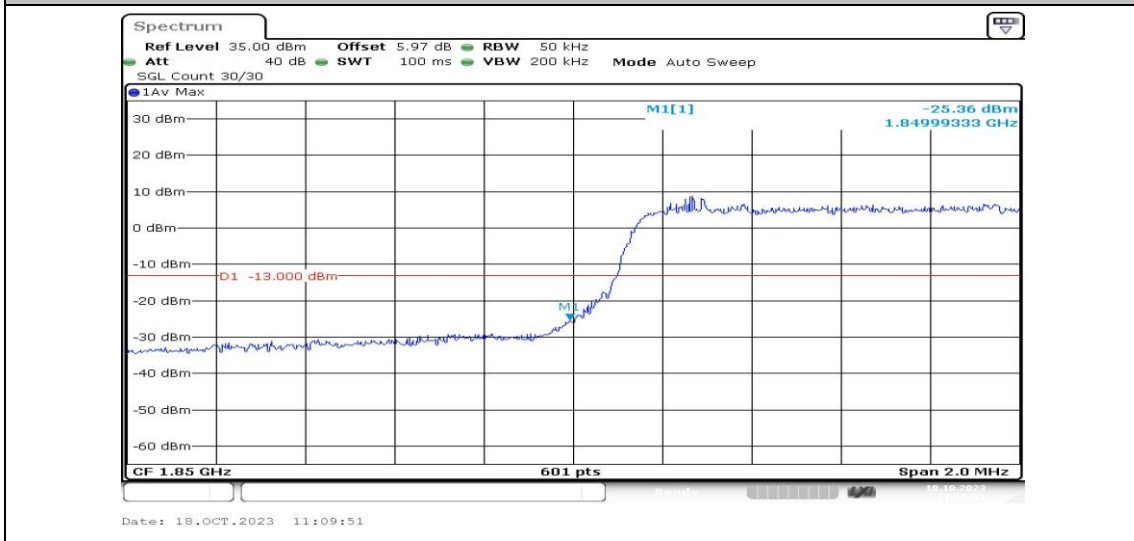
Band2-3MHz-QPSK-18615-15RB#0-PASS
