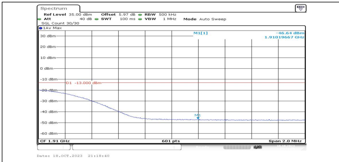
Band2-20MHz-QPSK-19100-1RB#0-PASS
