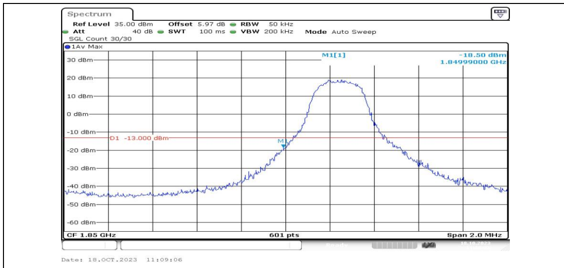
Band2-3MHz-QPSK-18615-1RB#0-PASS
