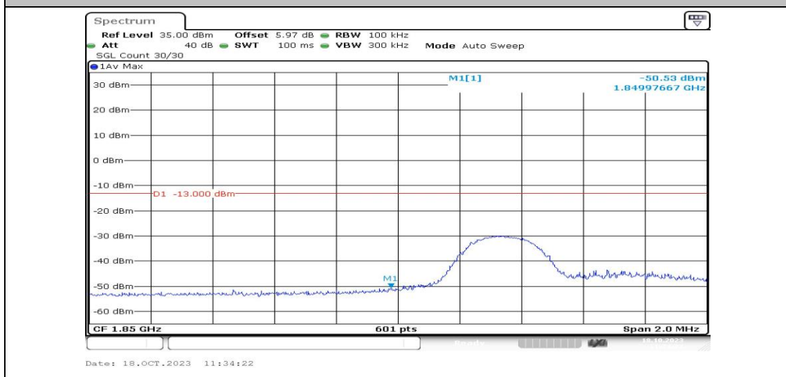
Band2-5MHz-QPSK-18625-1RB#24-PASS
