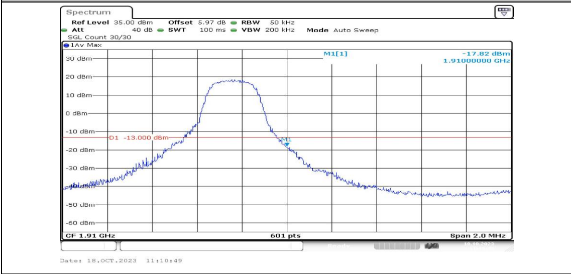
Band2-3MHz-QPSK-19185-1RB#14-PASS
