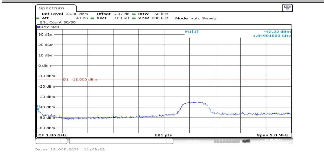
Band2-3MHz-QPSK-18615-1RB#14-PASS
