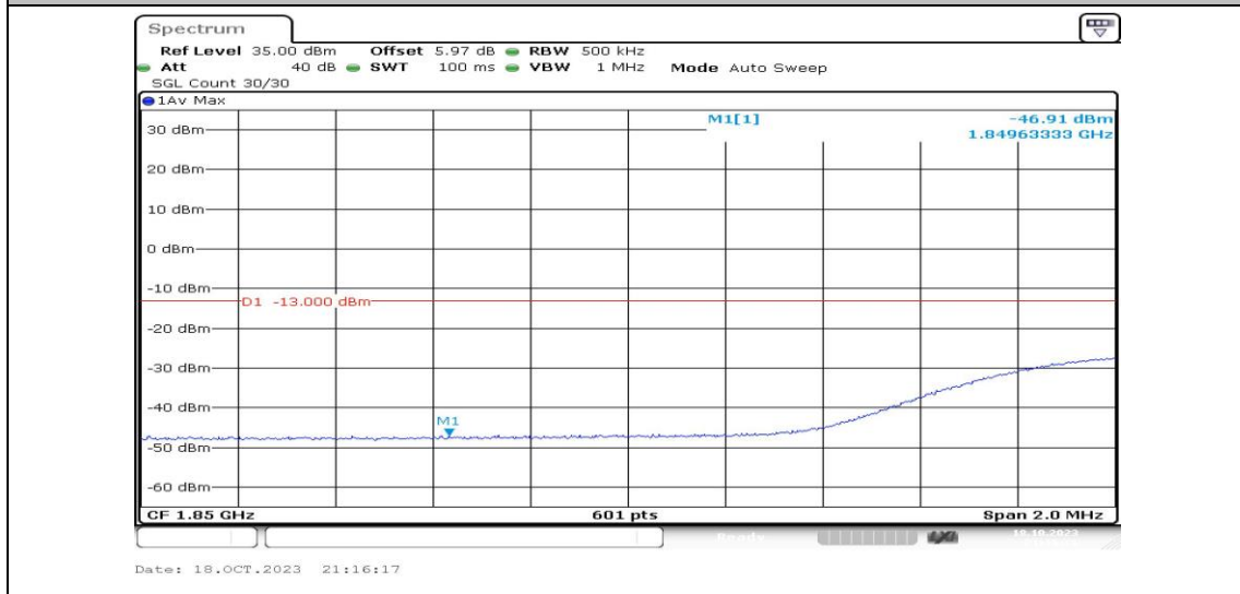
Band2-20MHz-QPSK-18700-1RB#99-PASS
