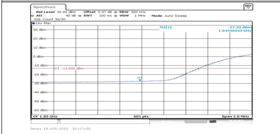
Band2-20MHz-QPSK-18700-100RB#0-PASS
